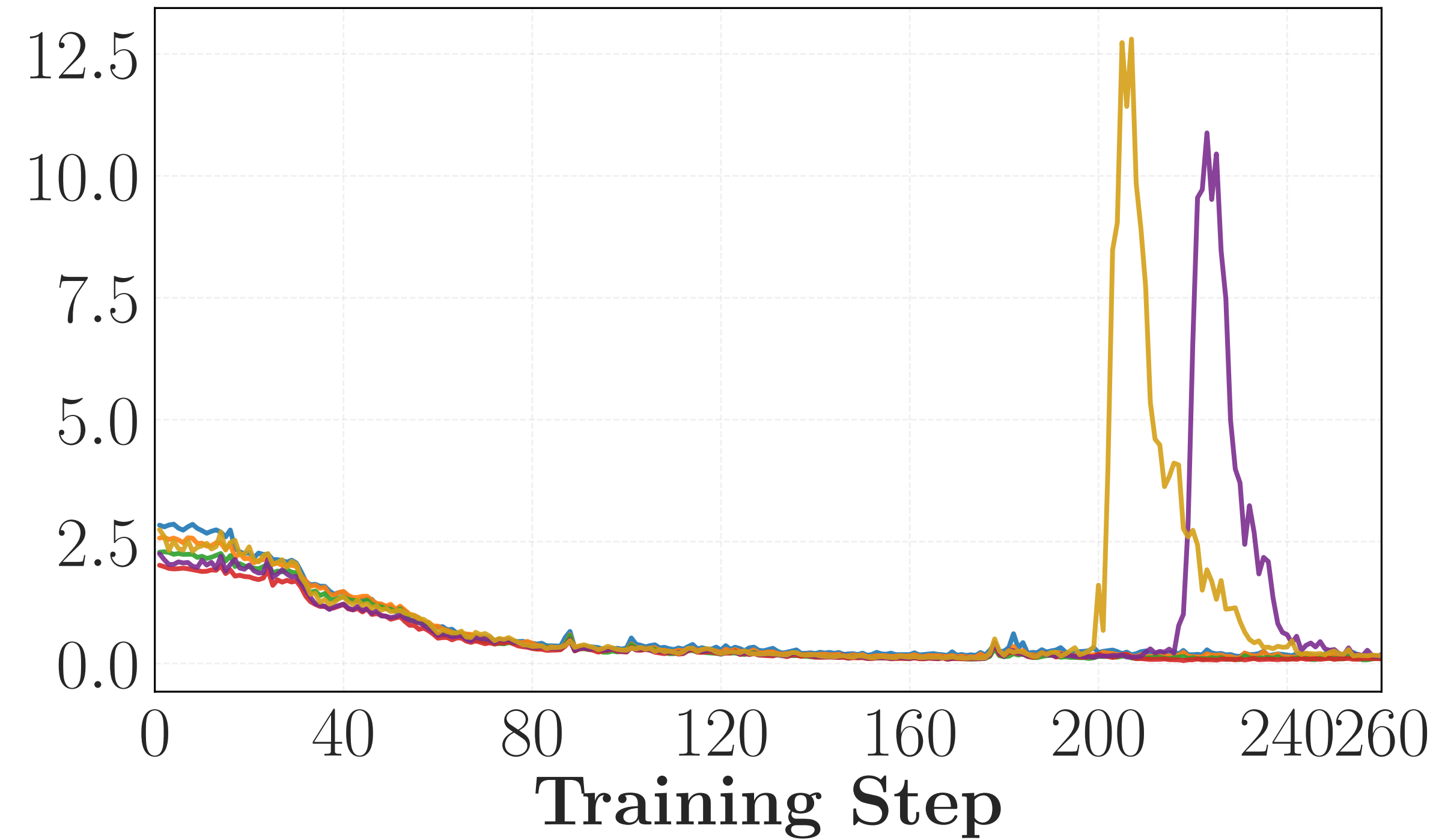
Grad Norm
