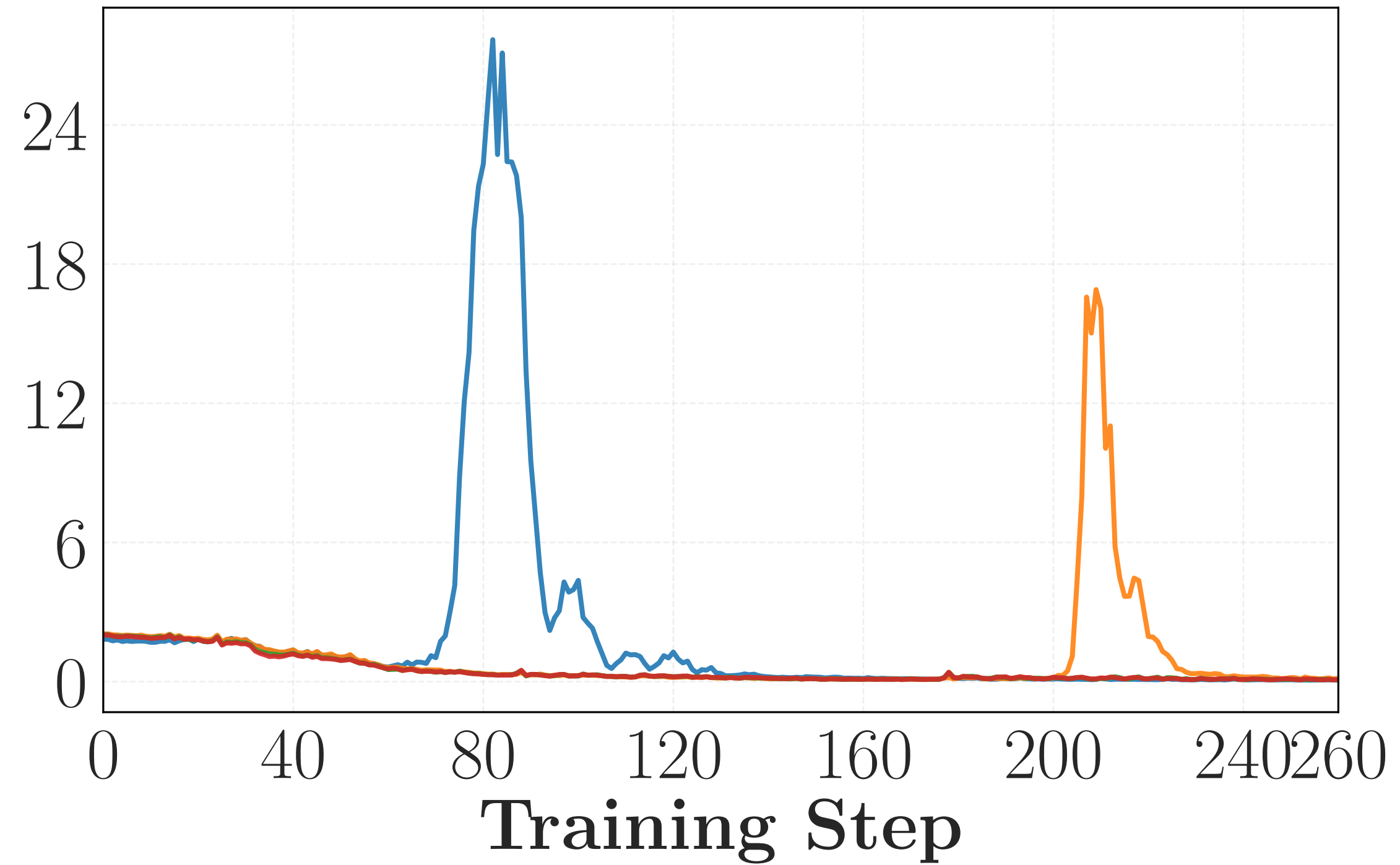
Grad Norm
