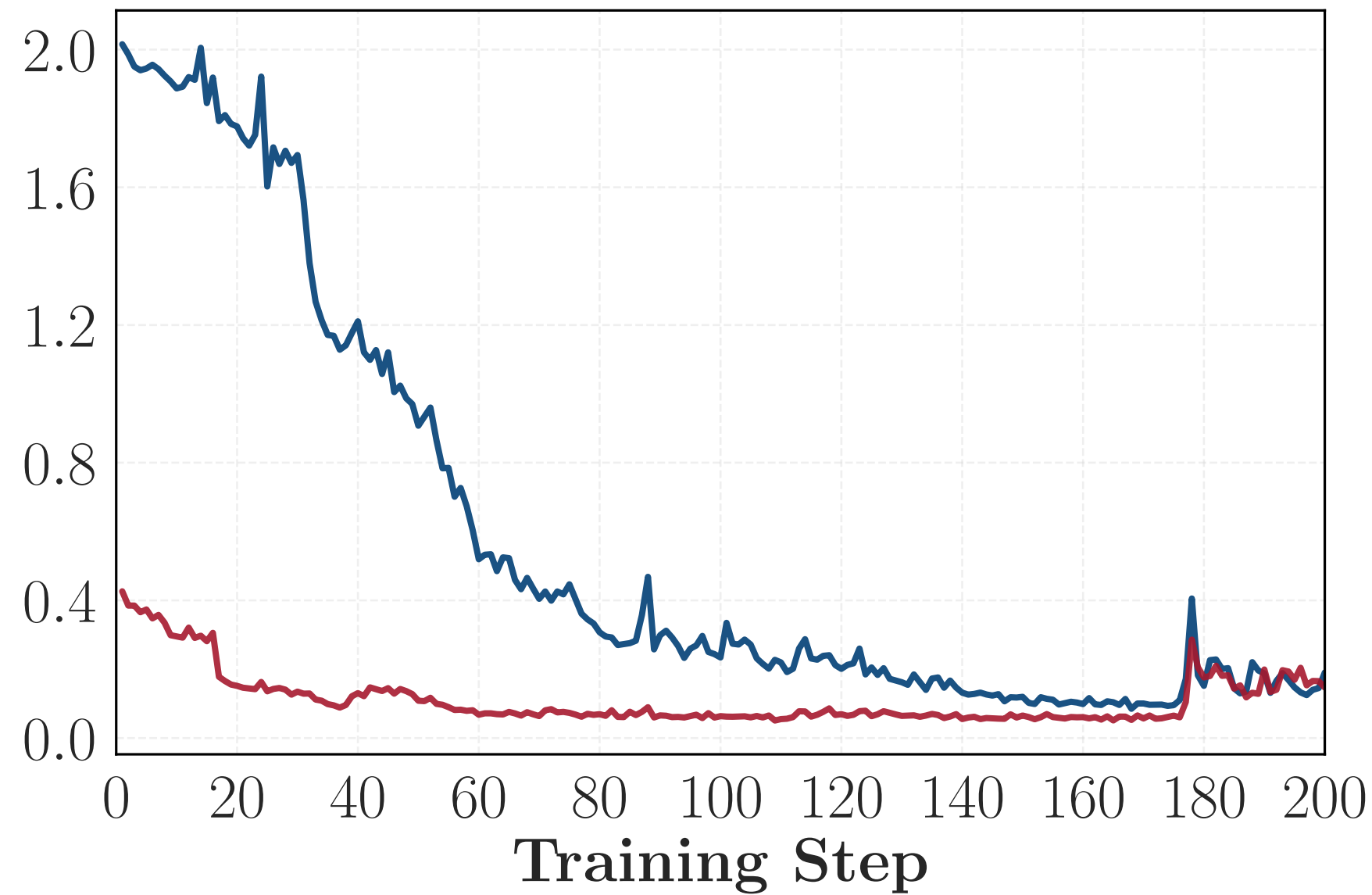
Grad Norm
