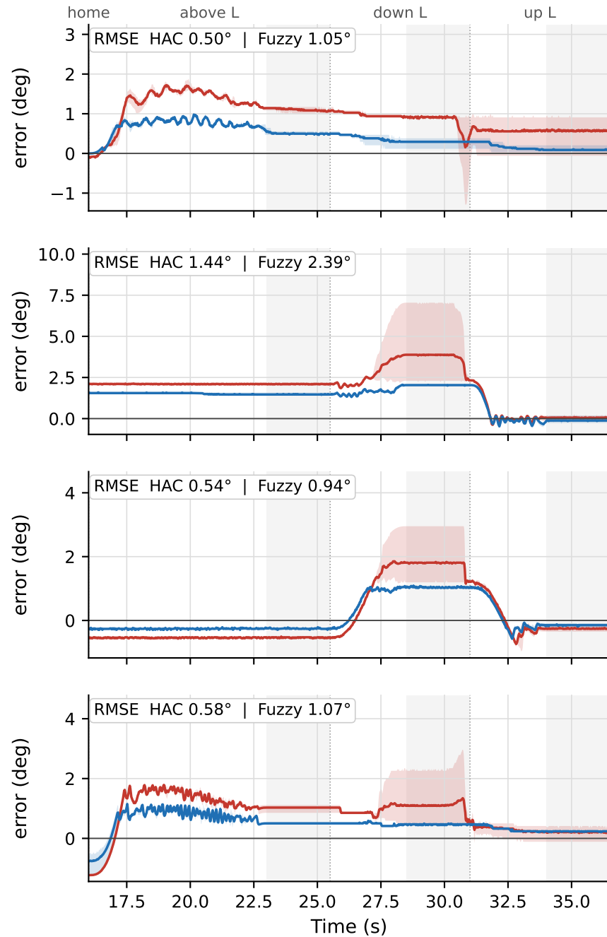
Tracking error
