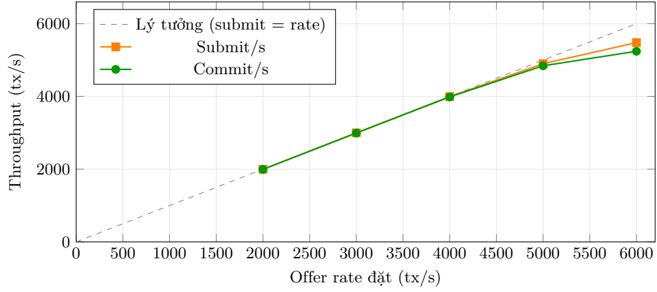
Fig. 14. Ed25519: pipeline bám offer rate tới 4k tx/s; bảo hòa nhẹ từ 5k với commit \sim 4,8\text{--}5,2\text{k tx/s} .
