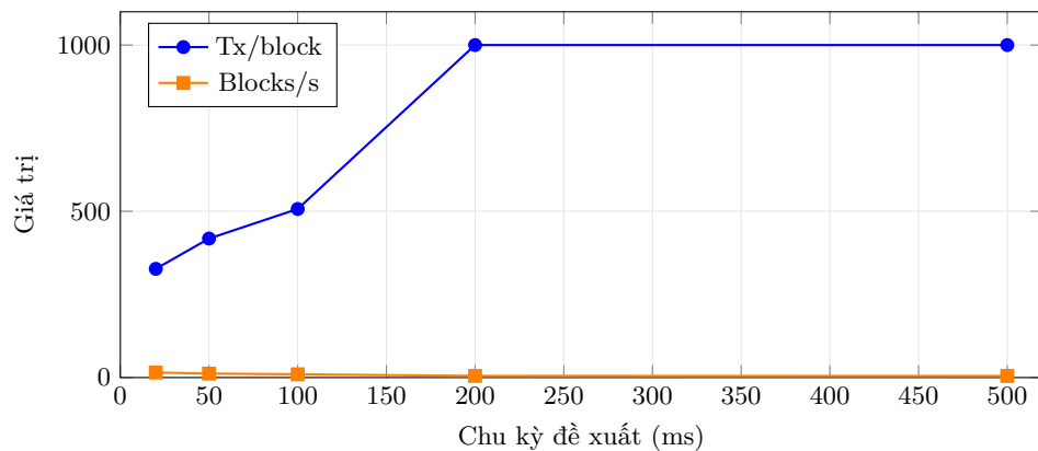
Fig. 11. Ở tải 5.000 tx/s: chu kỳ ngắn cho nhiều block nhỏ, chu kỳ dài cho ít block lớn (bão hòa ở kích thước lô 1.000); thông lượng commit không đổi \sim 5.000 tx/s.
