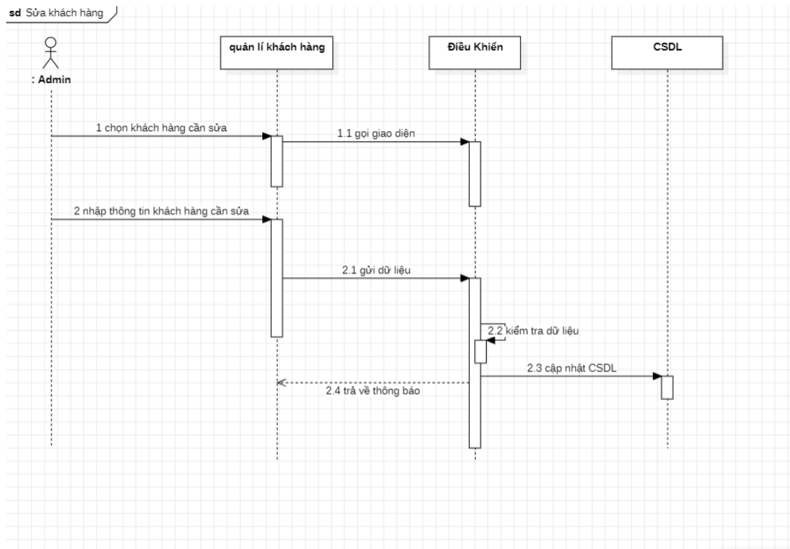
Figure 3-11: Sơ đồ tuần tự sửa khách hàng.
