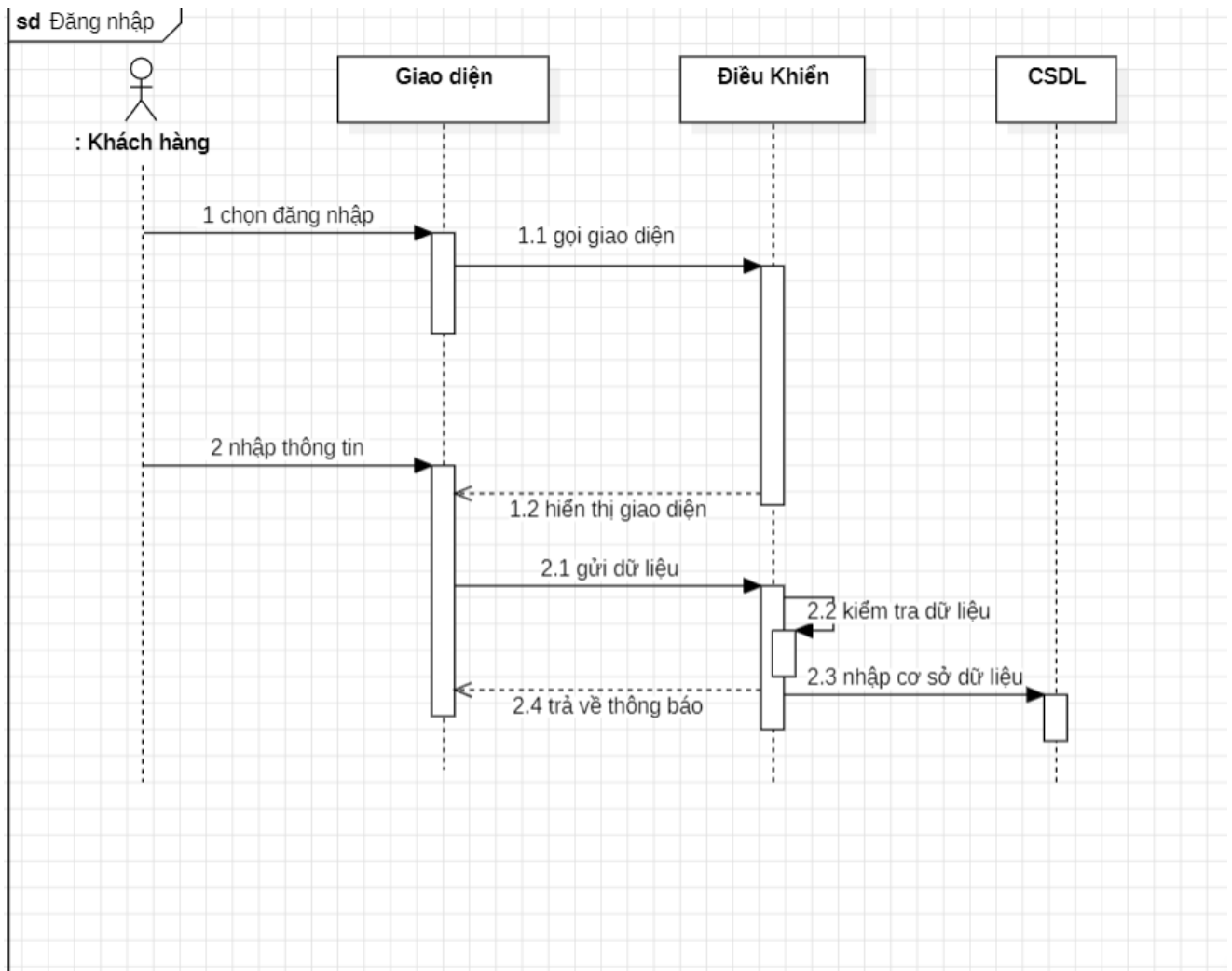
Figure 3-8: Sơ đồ tuần tự đăng nhập.
