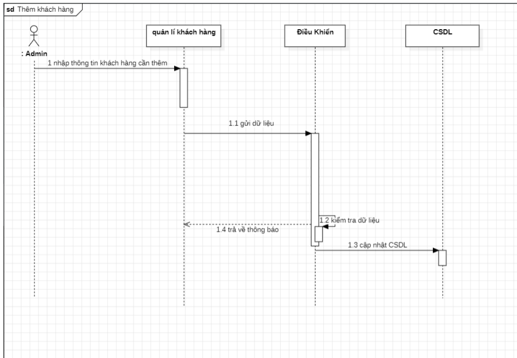
Figure 3-13: Sơ đồ tuần tự thêm khách hàng.
