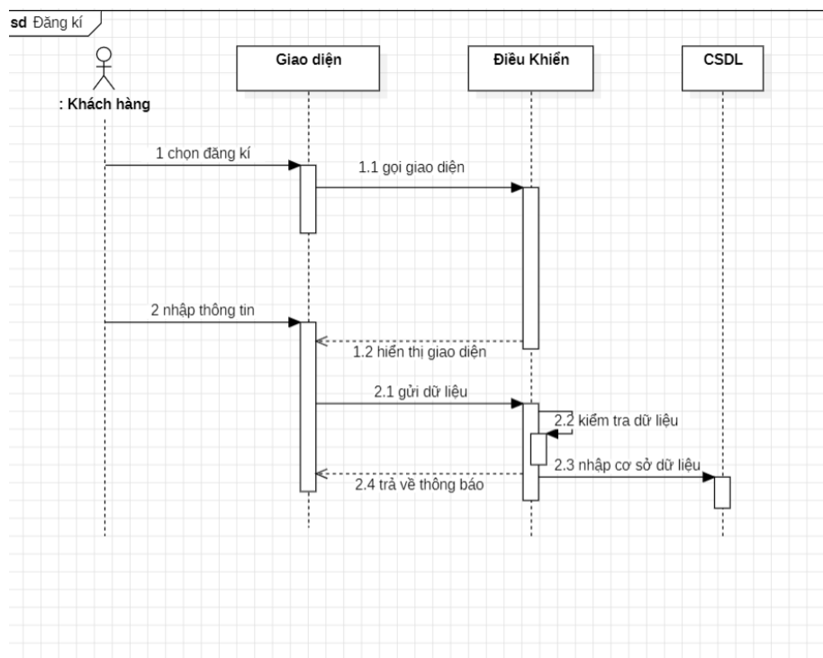
Figure 3-9: Sơ đồ tuần tự đăng kí.
