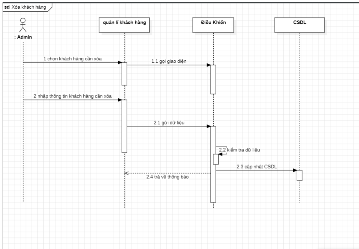
Figure 3-12: Sơ đồ tuần tự xóa khách hàng.
