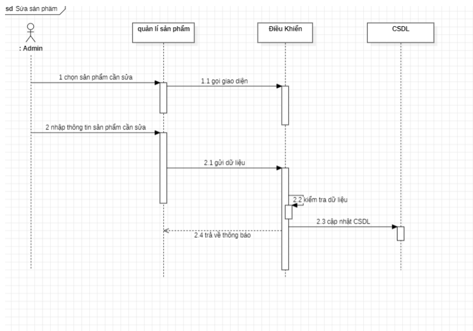
Figure 3-5: Sơ đồ tuần tự sửa sản phẩm.
