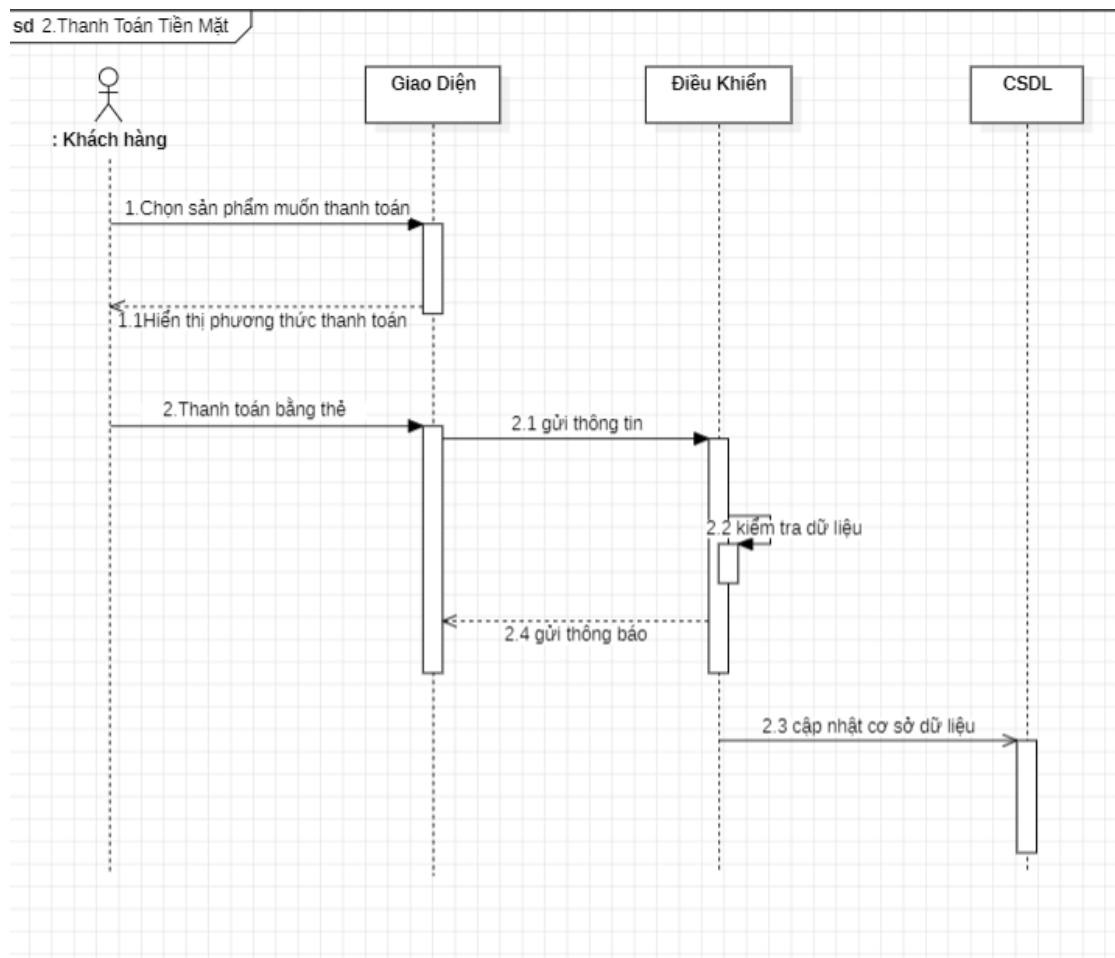
Figure 3-2: Sơ đồ tuần tự thanh toán tiền mặt.
