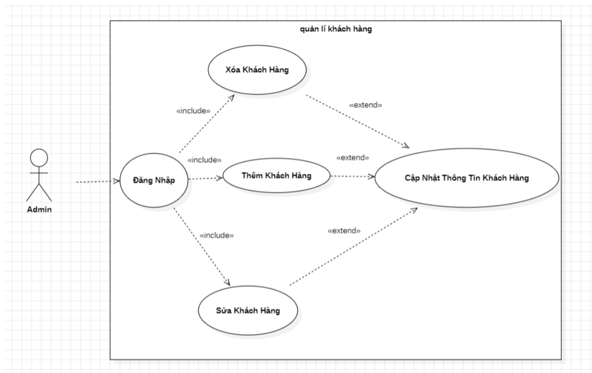
Figure 3-10: Sơ đồ chức năng quản lí khách hàng
