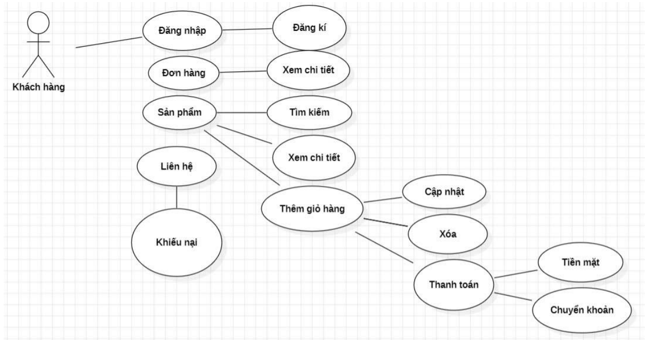
Figure 2-3: Usecase khách hàng.
