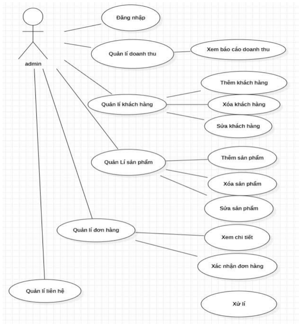
Figure 2-2: Usecase Tổng quát.
