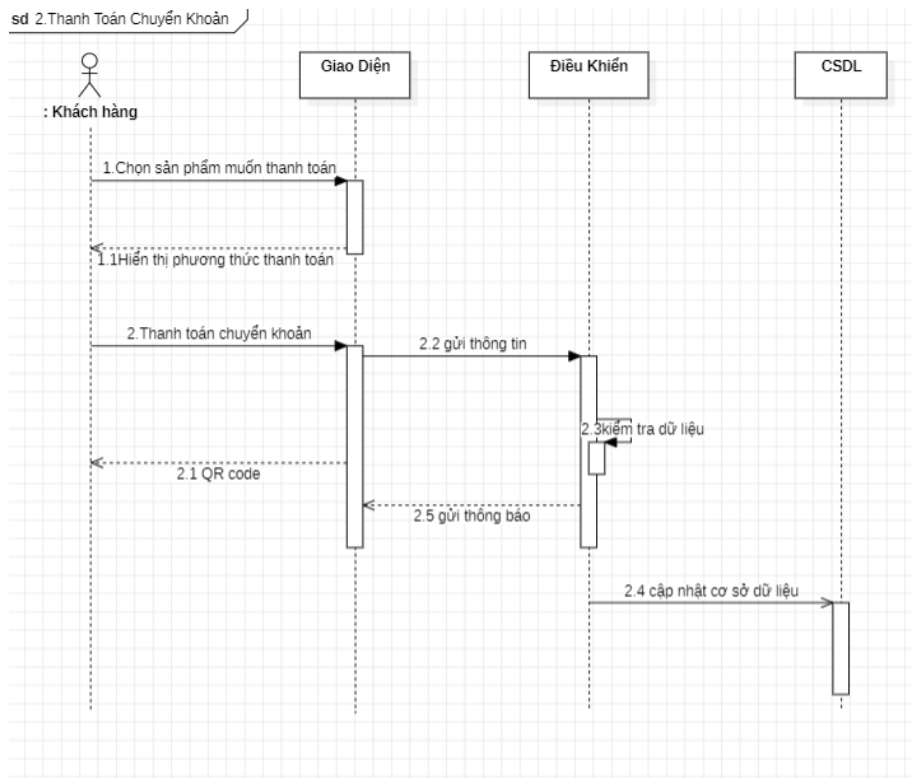
Figure 3-3: Sơ đồ tuần tự thanh toán chuyển khoản.
