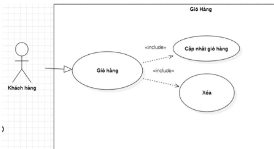
Figure 3-14: Sơ đồ chức năng giỏ hàng.
