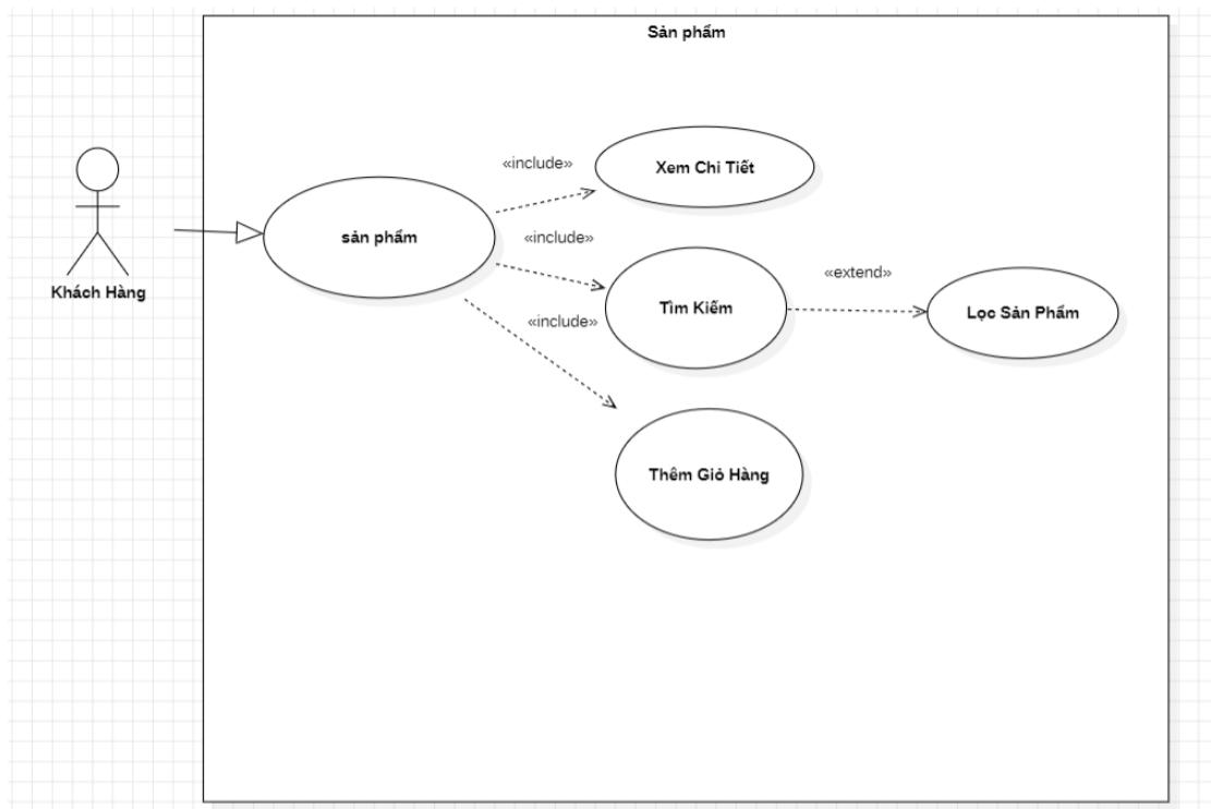
Figure 3-15: Sơ đồ chức năng sản phẩm.
