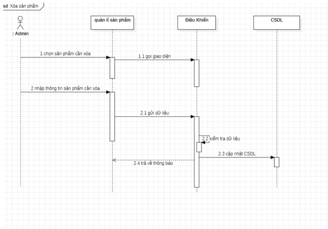
Figure 3-6: Sơ đồ tuần tự xóa sản phẩm
