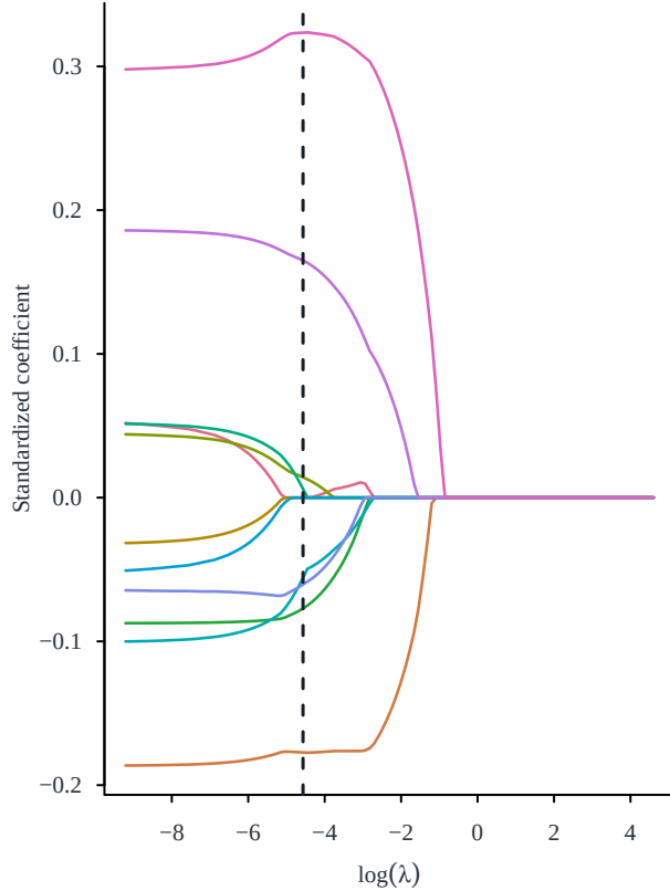
Lasso paths
