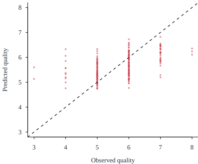
Lasso (RMSE 0.700)
