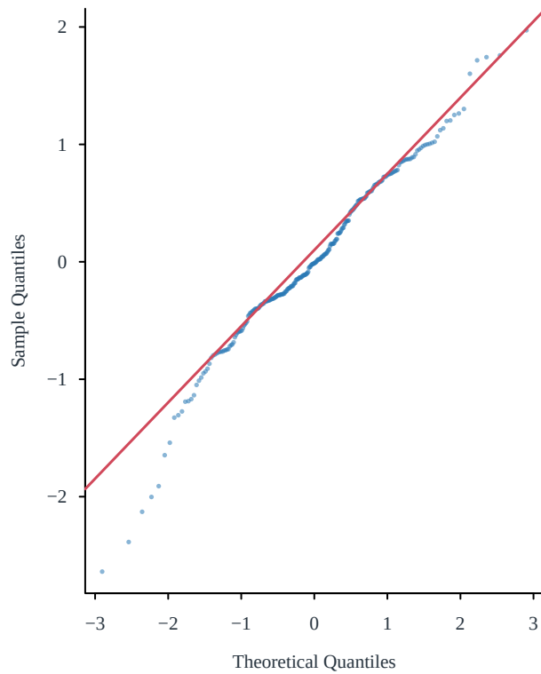
Normal Q-Q
