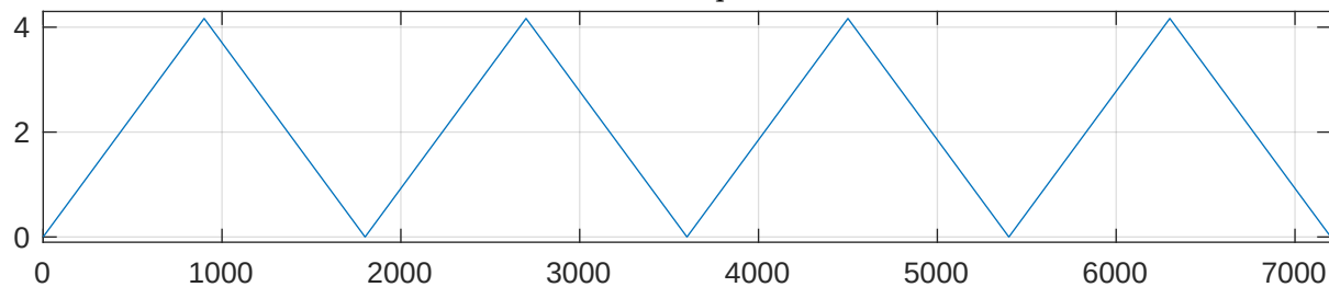
EGF input
