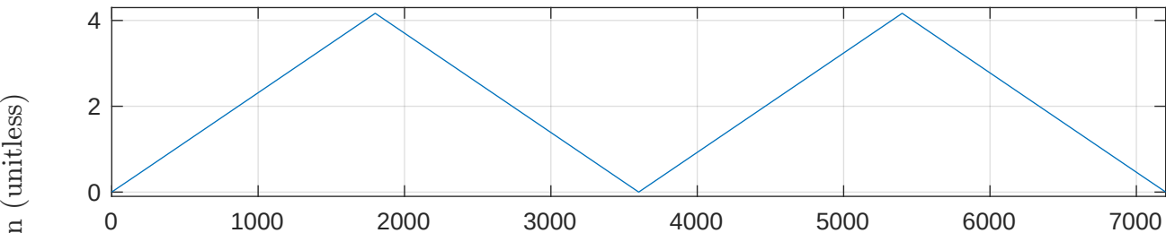
EGF input
