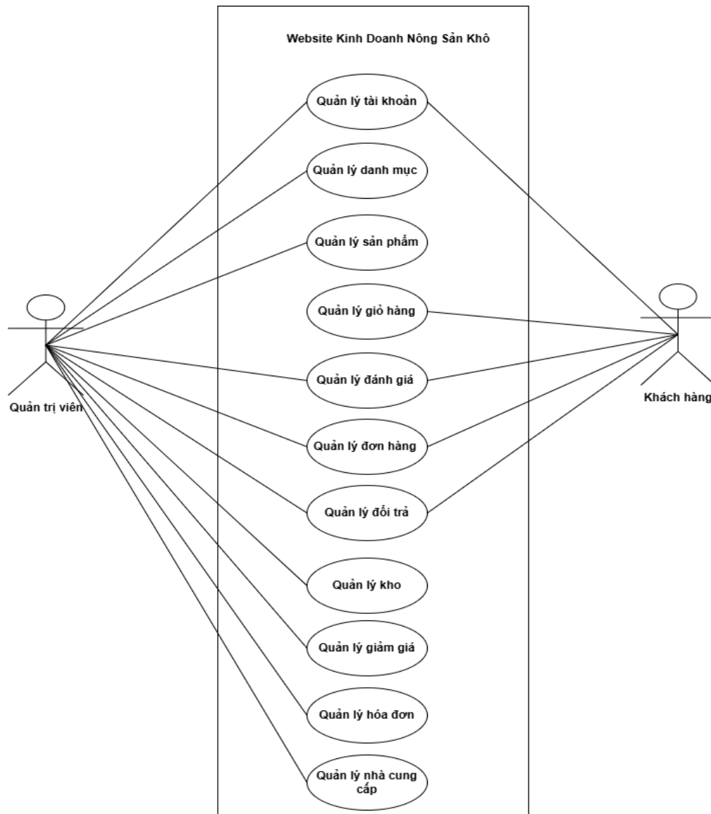
Hình 2-75: Sơ đồ Use case tổng quát.
