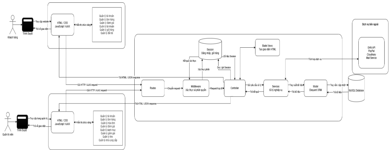
Hình 3-1: Sơ đồ kiến trúc tổng thể.
