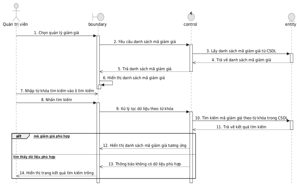
Hình 3-48: Sơ đồ tuần tự tìm kiếm giảm giá của quản trị viên.
