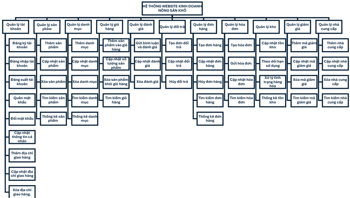
Hình 2-74: Sơ đồ chức năng.
