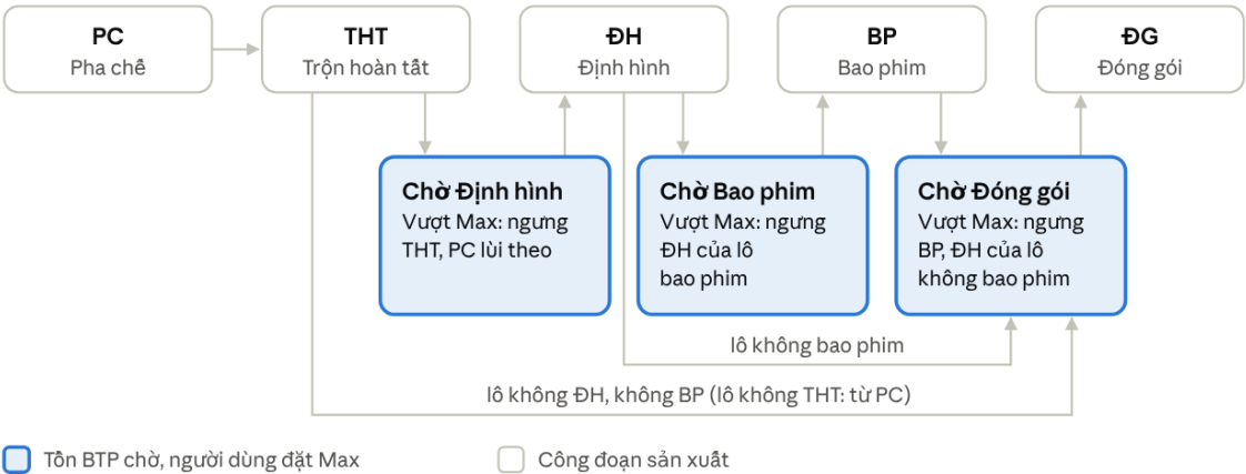
Hình 1. Dòng chảy công đoạn – 3 nhóm tồn BTP chờ
