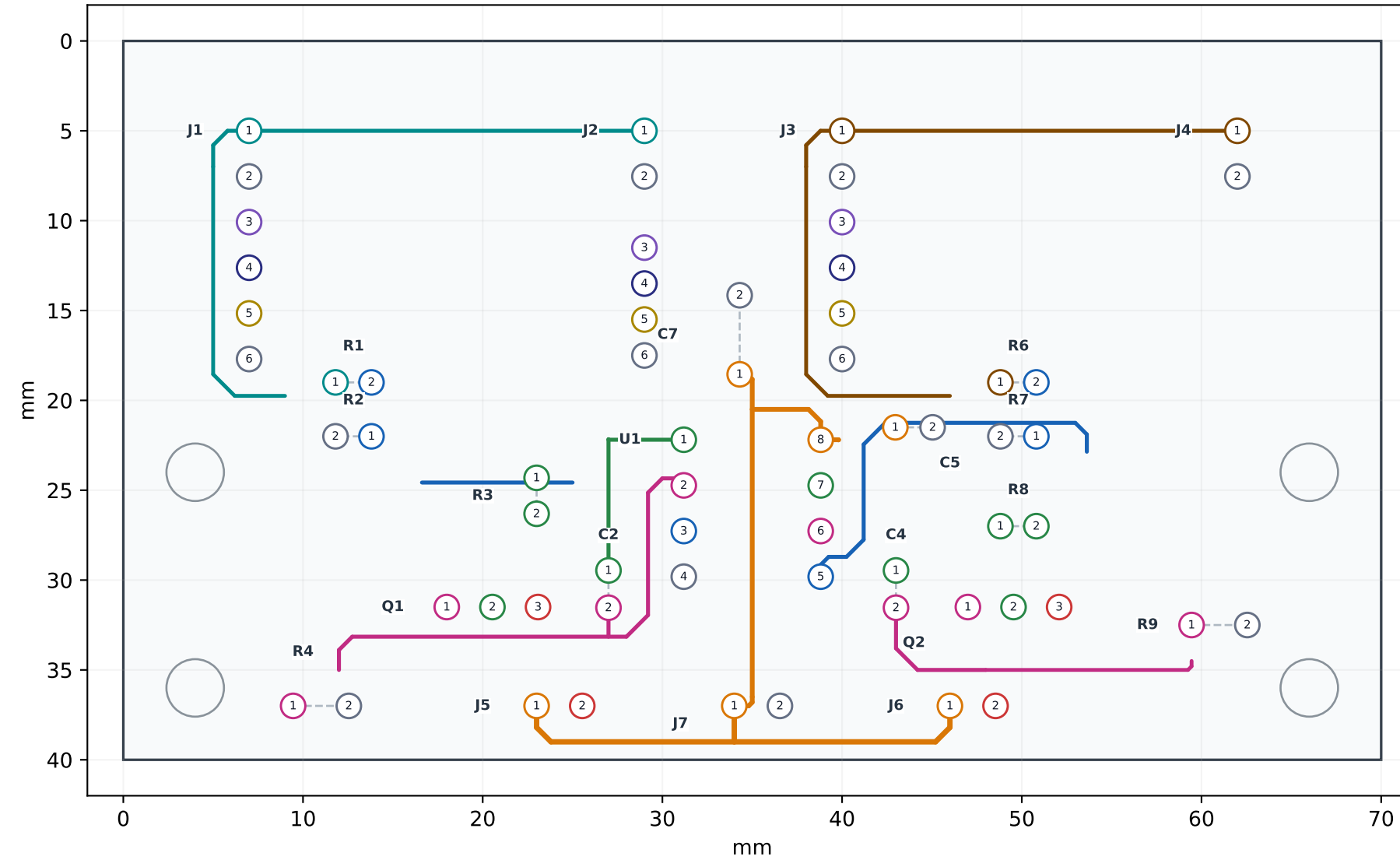
Mặt dưới — B.Cu (nhìn xuyên từ trên)
