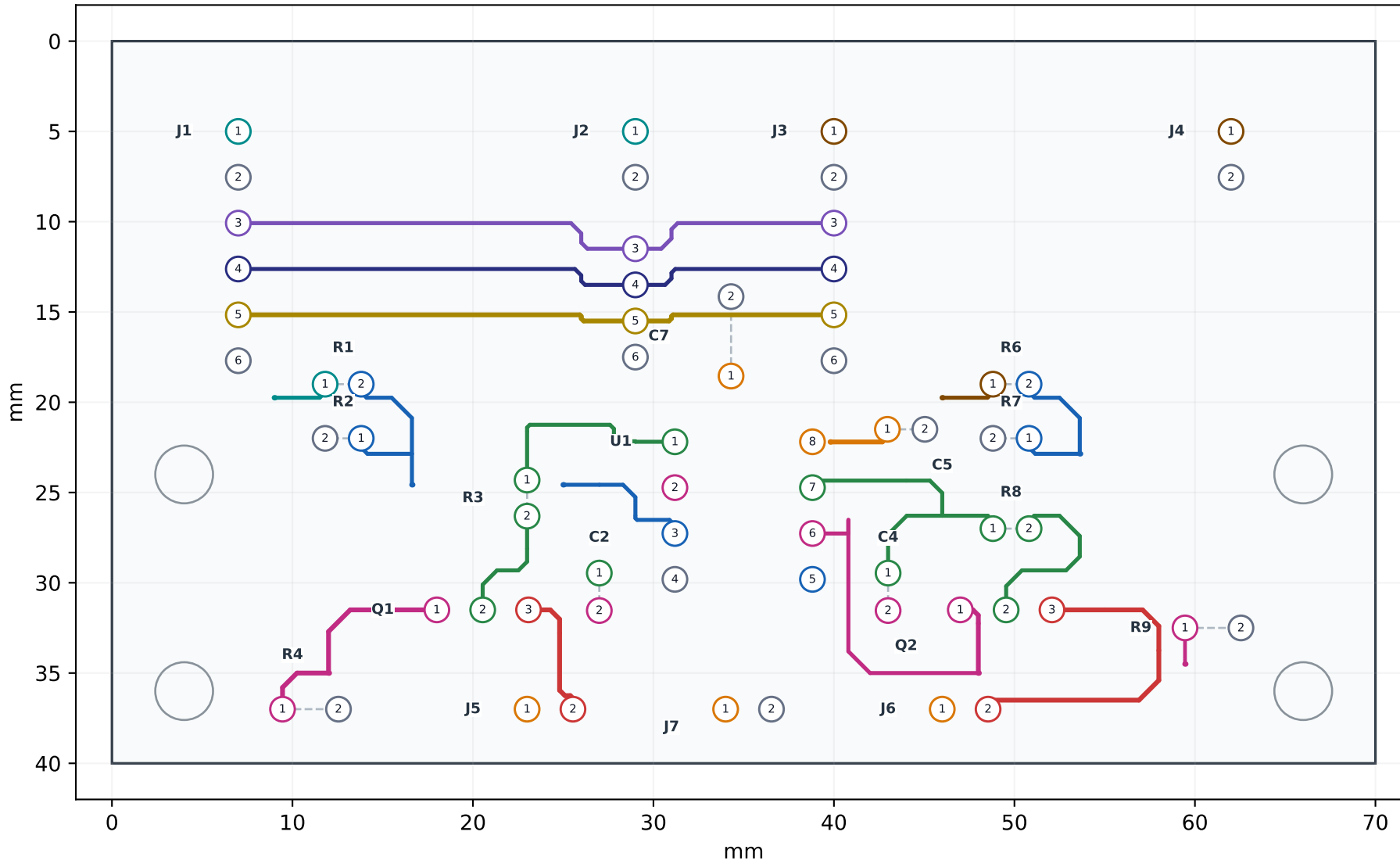
Mặt trên — F.Cu
