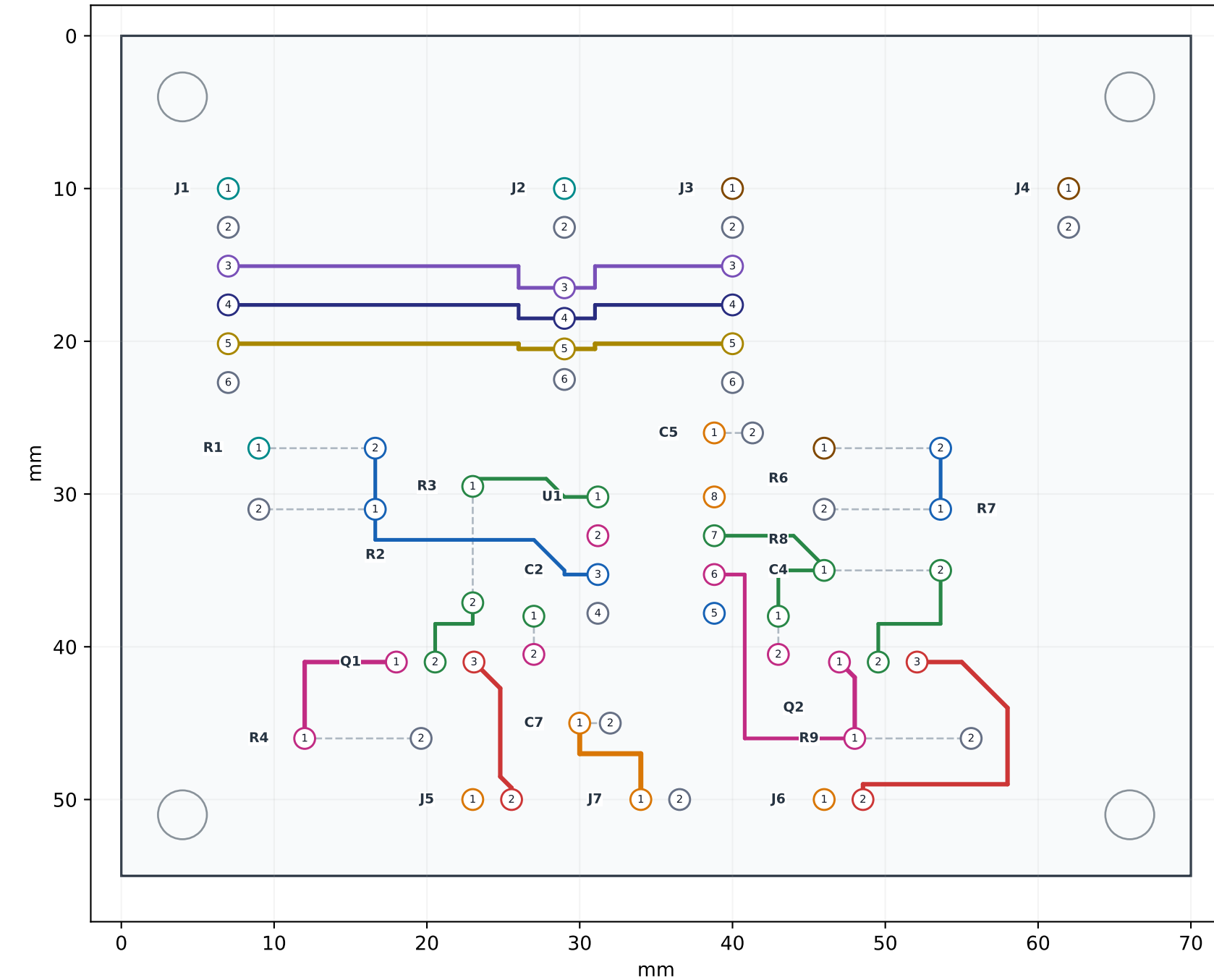
Mặt trên — F.Cu
