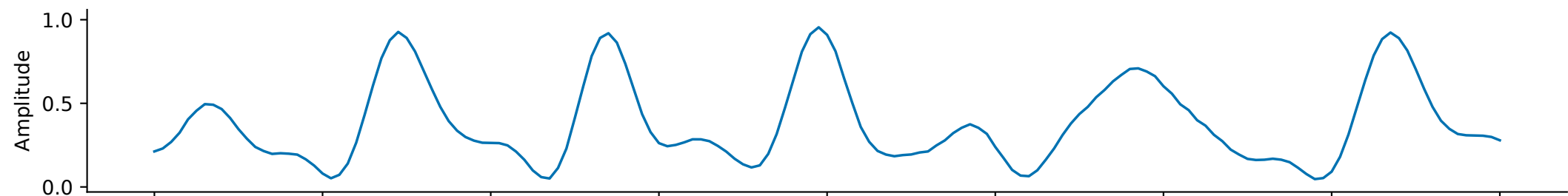
TCN-FiLM
