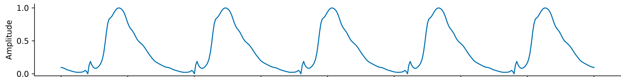
LSM-GAN
