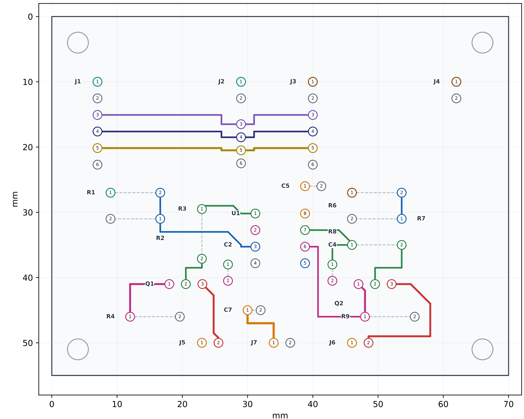
Mặt trên — F.Cu
