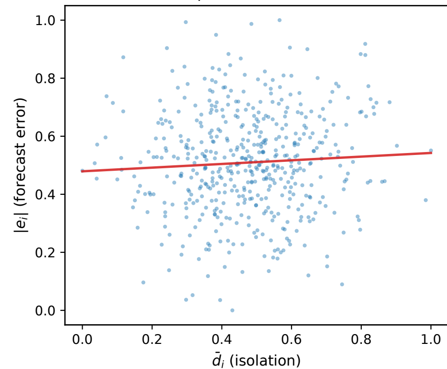
CSI800 \rho = 0.02 (n.s.)
