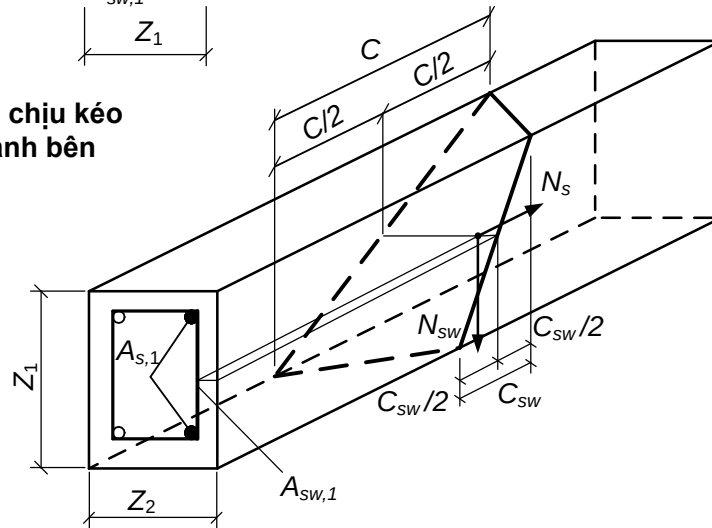
Hình 12 – Sơ đồ nội lực trong tiết diện không gian khi tính toán chịu mô men xoắn
