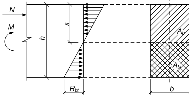
Hình 4 – Sơ đồ nội lực và biểu đồ ứng suất (tại trạng thái giới hạn) trong tiết diện thẳng góc với trục dọc cầu kiện bê tông chịu uốn (chịu nén lệch tâm) khi tính toán độ bền có kể đến cường độ chịu kéo của bê tông vùng chịu kéo
