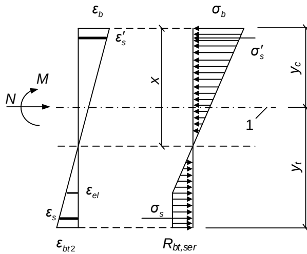
b) Dưới tác dụng của mô men và lực dọc
