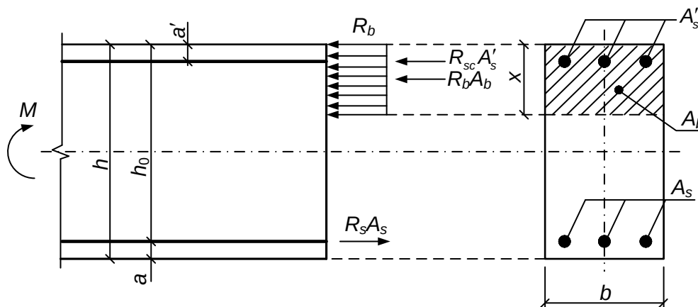
Hình 5 – Sơ đồ nội lực và biểu đồ ứng suất trong tiết diện thẳng góc với trục dọc cầu kiện bê tông cốt thép chịu uốn khi tính toán theo độ bền
