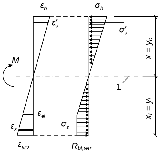
a) Dưới tác dụng của mô men
