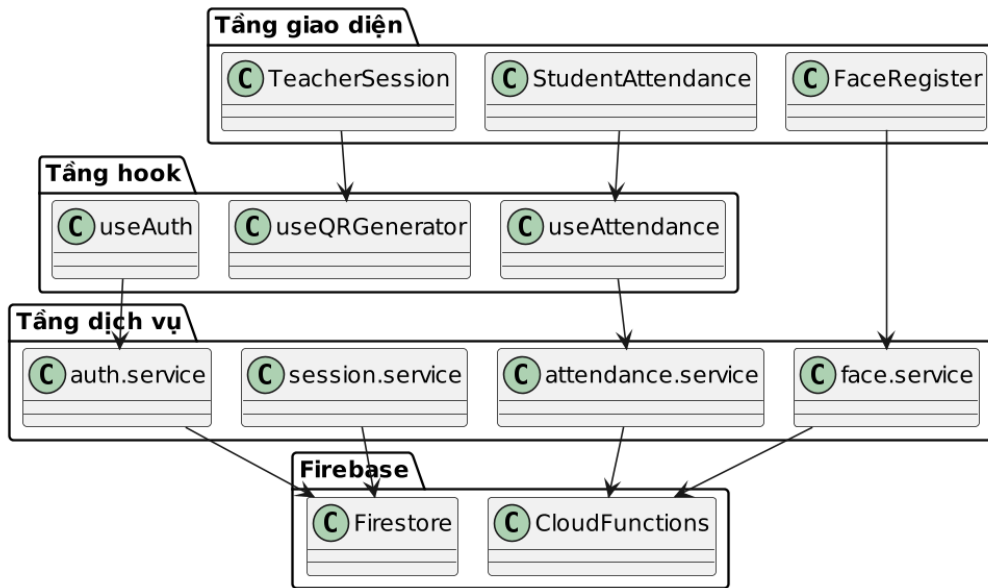
Hình 4.10: Sơ đồ phân lớp các thành phần phần mềm của Mini App
