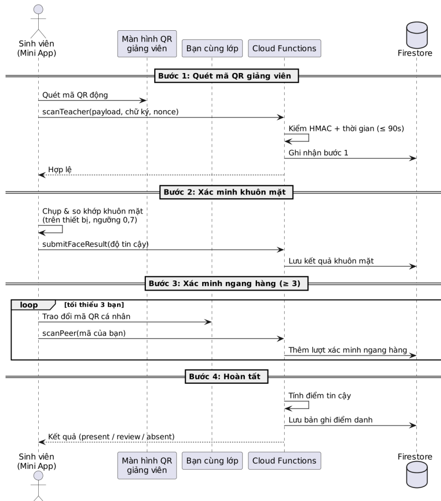
Hình 4.6: Lược đồ tuần tự quy trình điểm danh bốn bước
