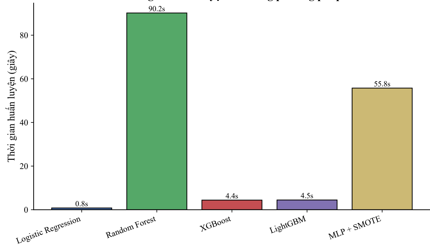
Thời gian huấn luyện của từng phương pháp
