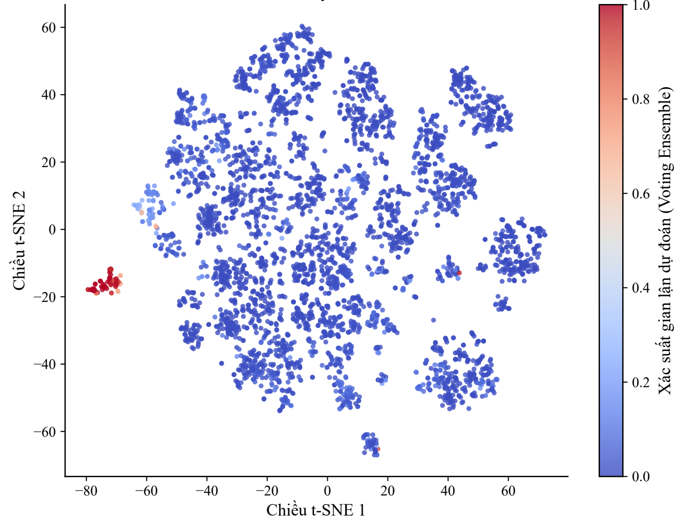
t-SNE theo xác suất dự đoán của Ensemble
