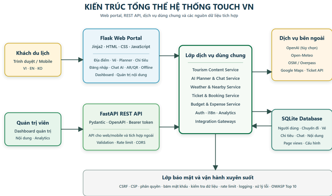
Hình 1. Kiến trúc Flask/FastAPI, lớp dịch vụ dùng chung, cơ sở dữ liệu và tích hợp ngoài.
