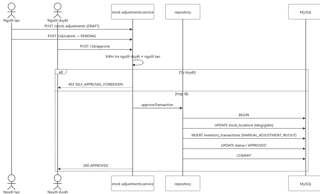
Hình 3-30: Sơ đồ tuần tự – Điều chỉnh tồn
