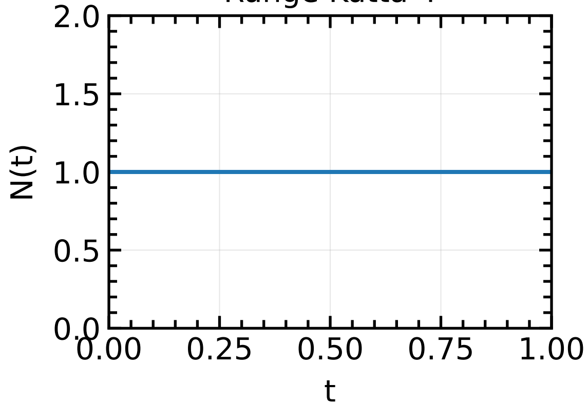
Runge Kutta 4
