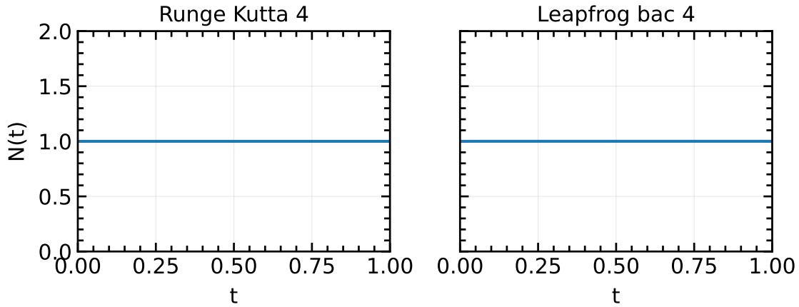
Figure 2: Chuẩn xác suất N(t) của RK4 và Leapfrog bậc 4. Hai ô dùng chung giới hạn trục tung.
