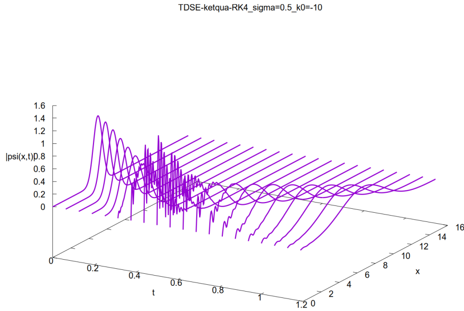
Figure 3: RK4 với \sigma_0 = 0.5 và k_0 = -10 : bó sóng truyền về phía -x , phản xạ ở biên trái rồi đổi chiều.
