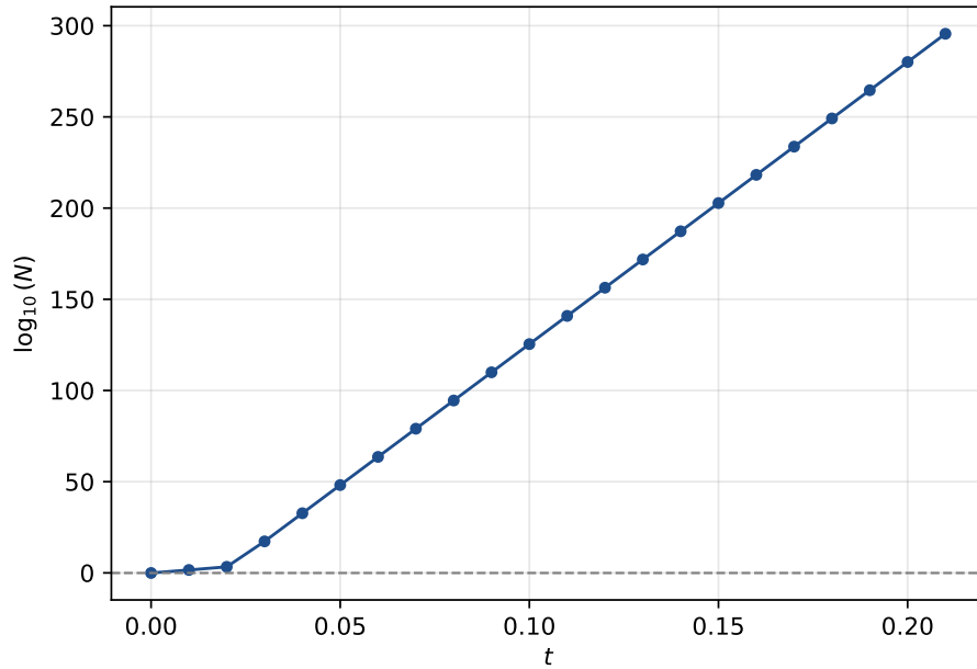
Hình 1: \log_{10} N(t) theo thời gian. Chuẩn hóa tăng từ \sim 0.886 lên hơn 10^{295} chỉ trong 0.21 đơn vị thời gian, và tràn số (inf) tại t = 0.22 .
