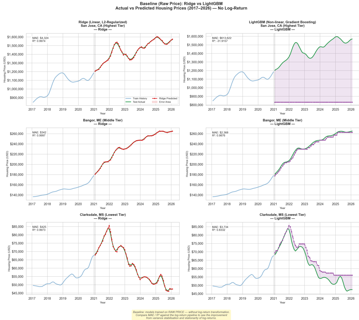
Hình 8: Đường cơ sở truyền thống — Ridge và LightGBM huấn luyện trực tiếp trên giá nhà thô (USD), không sử dụng biến đổi log-return, trên 3 phân khúc thị trường đại diện
