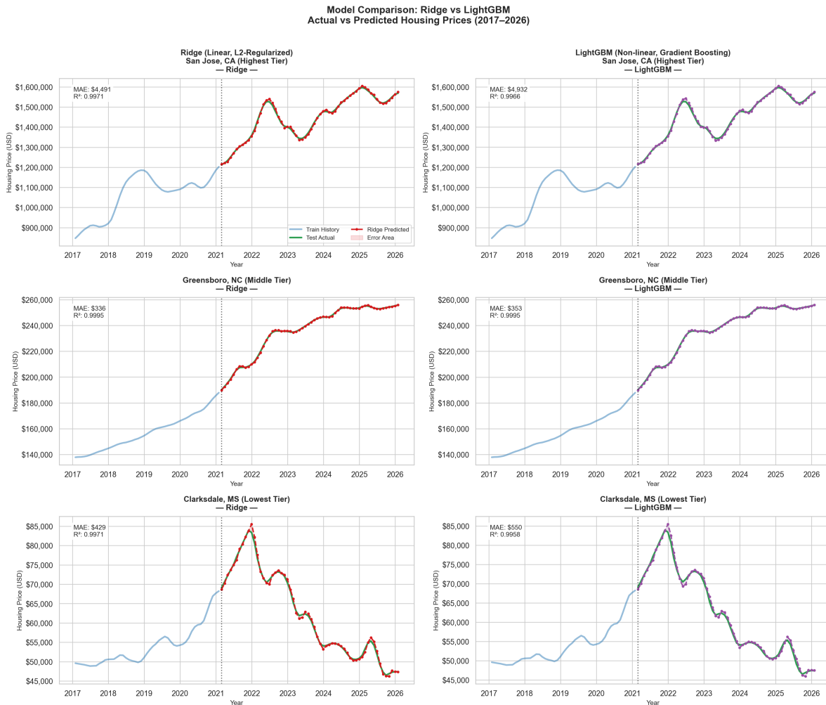
Hình 9: Giá nhà thực tế so với giá dự báo của Ridge (trái) và LightGBM (phải) trên 3 phân khúc thị trường đại diện
