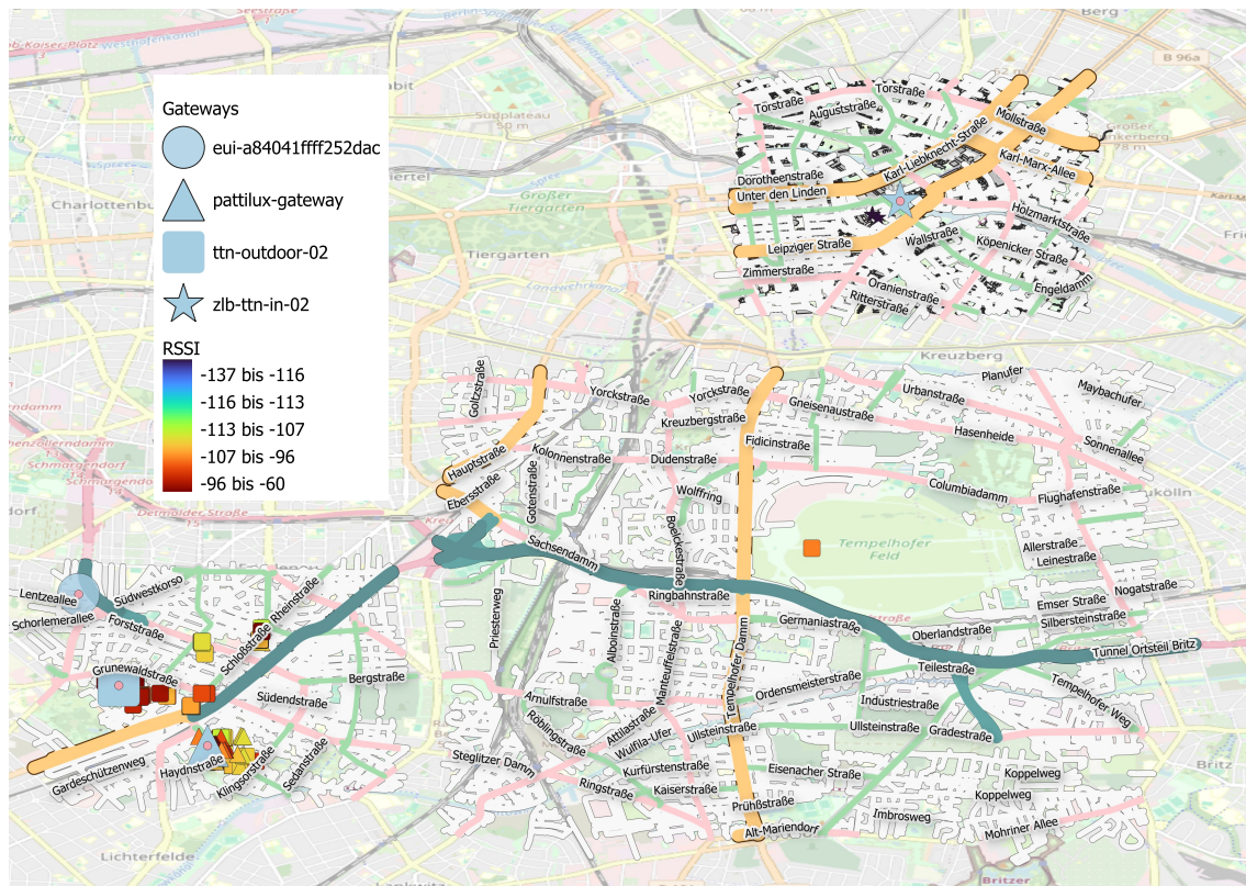
Abbildung 5.2: Ergebnisse der Netzabdeckungsanalyse in Berlin.
