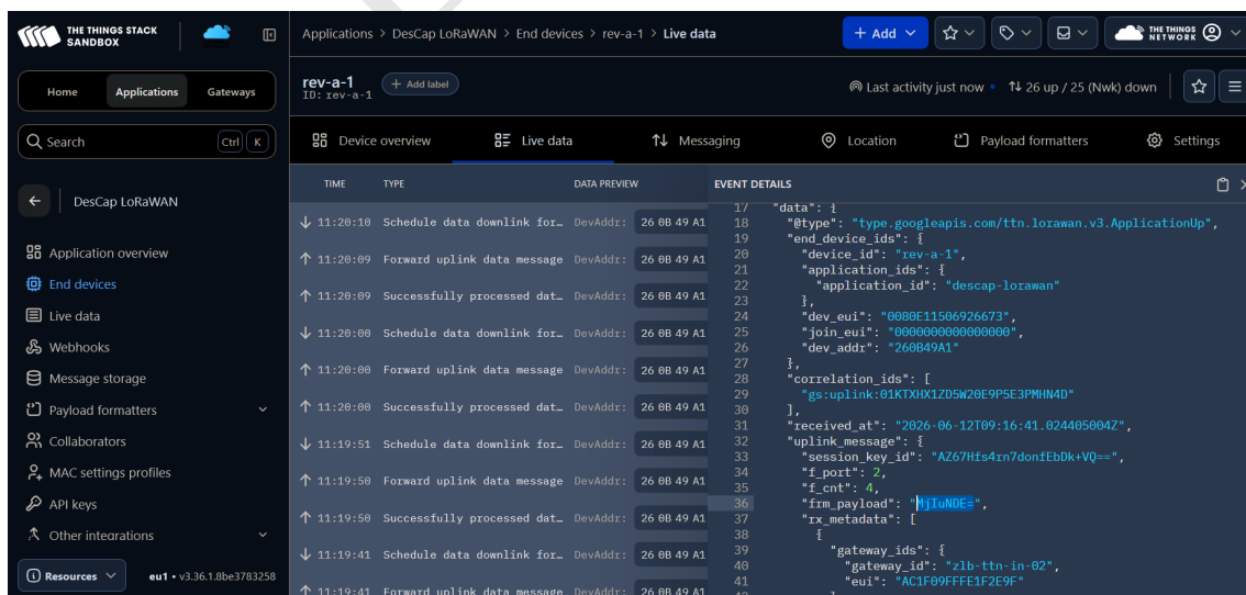
Abbildung 5.1: Screenshot von TTN-Konsole nach erfolgreichem Join-Request
