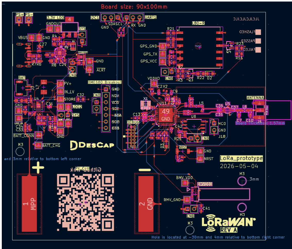
Abbildung 3.26: 2D-Ansicht der fertigen Leiterplatte
