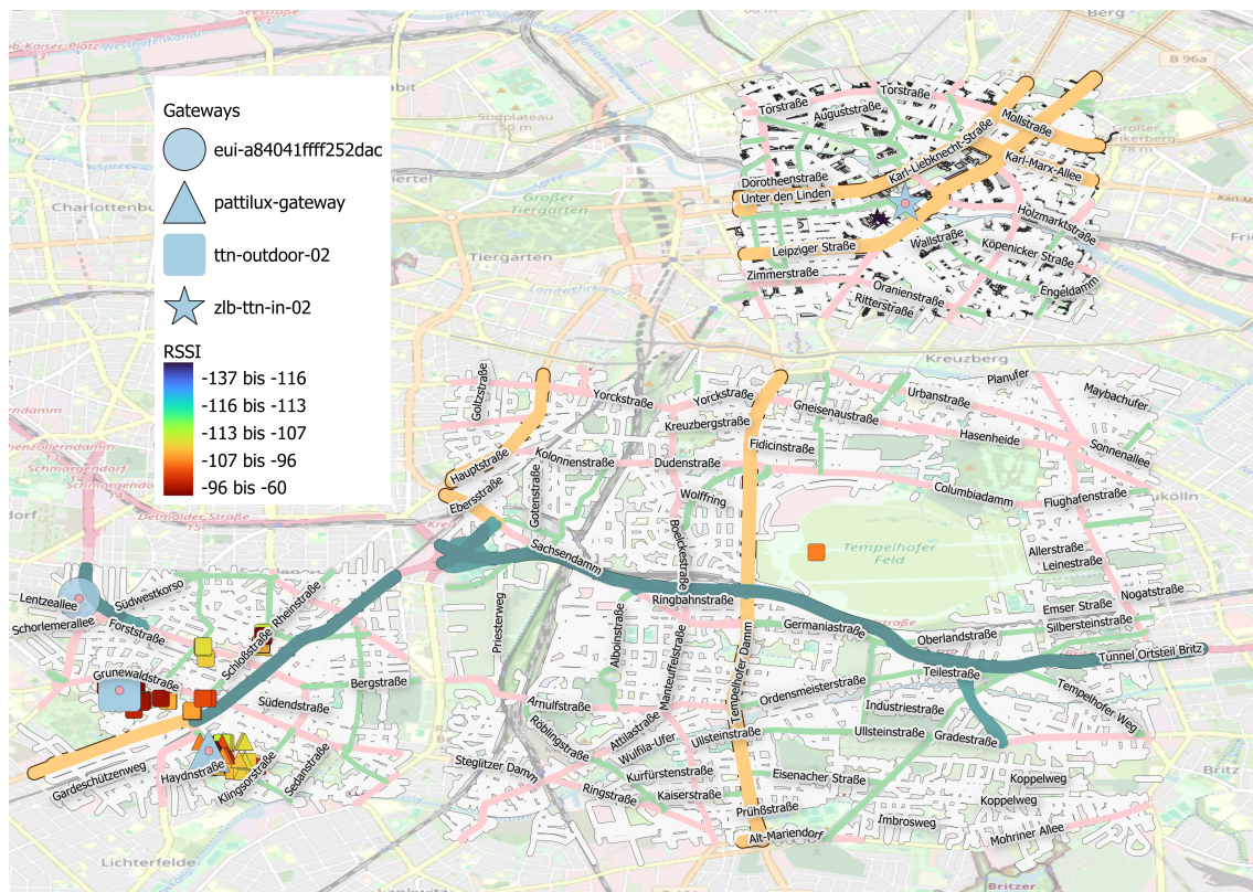
Abbildung 3.33: Ergebnisse der Netzabdeckungsanalyse in Berlin.
