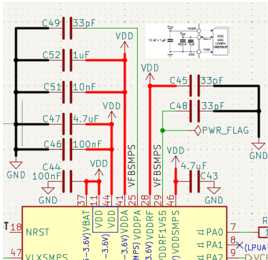
Abbildung 3.17: Entkopplungsschema der MCU
