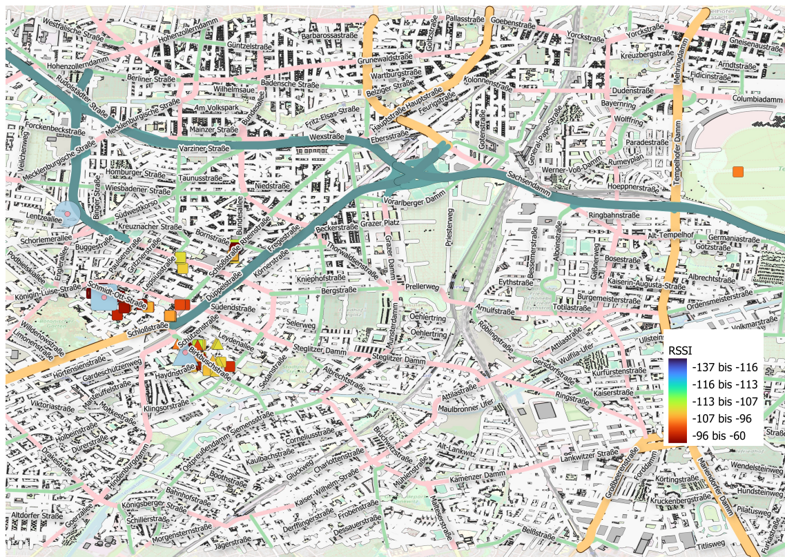
Abbildung 3.34: Netzabdeckungsanalyse in Steglitz und Tempelhof.
