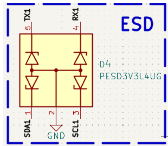
Abbildung 3.21: ESD-Schutz für Testheaders
