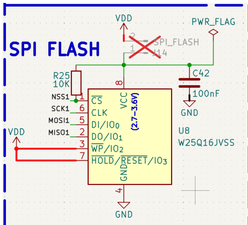
Abbildung 3.22: SPI-Flash-Speicher
