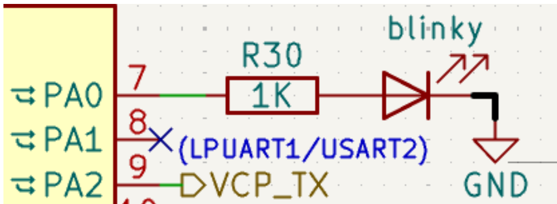
Abbildung 3.23: Status-LED
