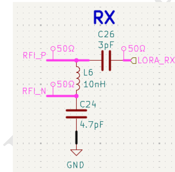
Abbildung 3.16: RX-Impedanzanpassung
