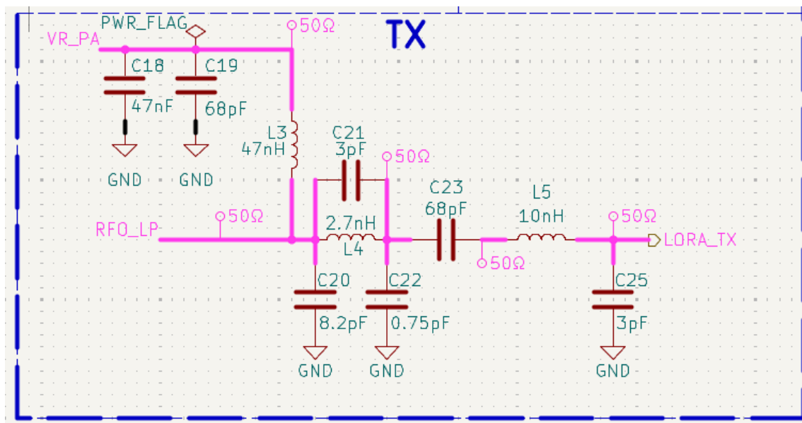
Abbildung 3.15: TX-Impedanzanpassung
