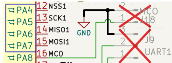
Abbildung 3.13: Überprüfung der TCXO-Frequenz über MCO-Ausgang
