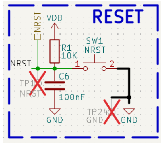
Abbildung 3.18: MCU-Reset-Schaltung
