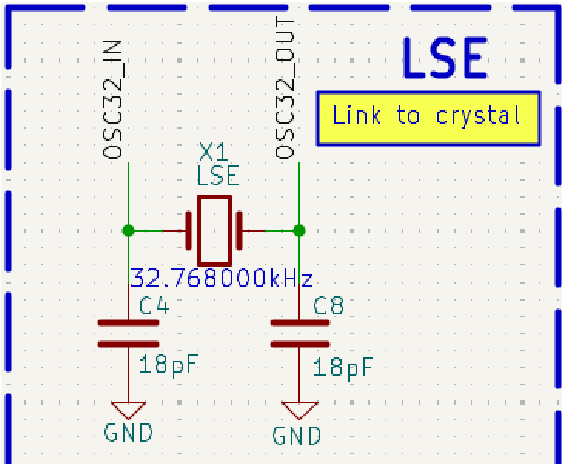
Abbildung 3.12: Taktversorgung mit LSE
