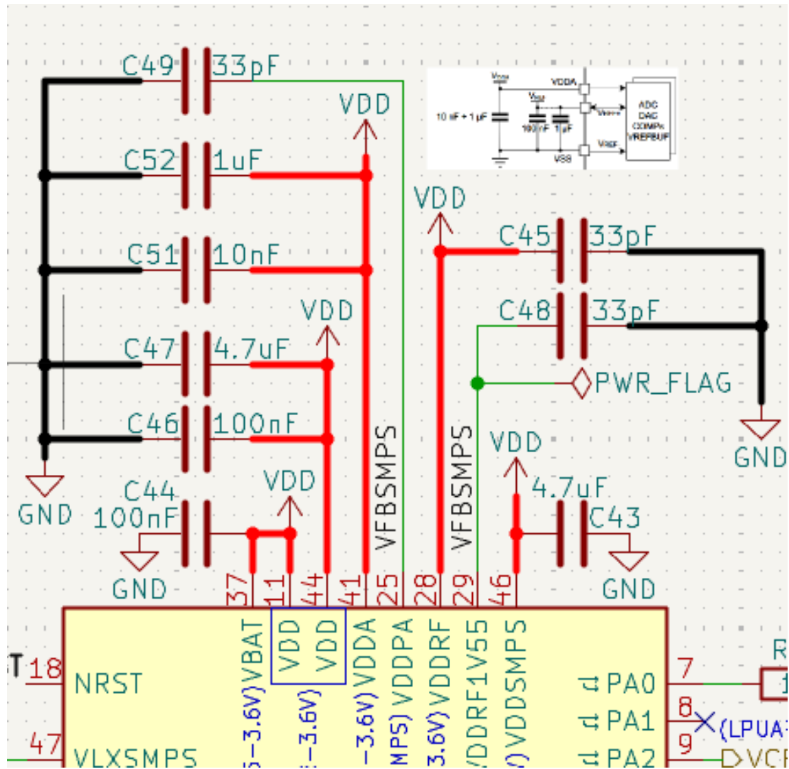
Abbildung 3.15: Entkopplungsschema der MCU
