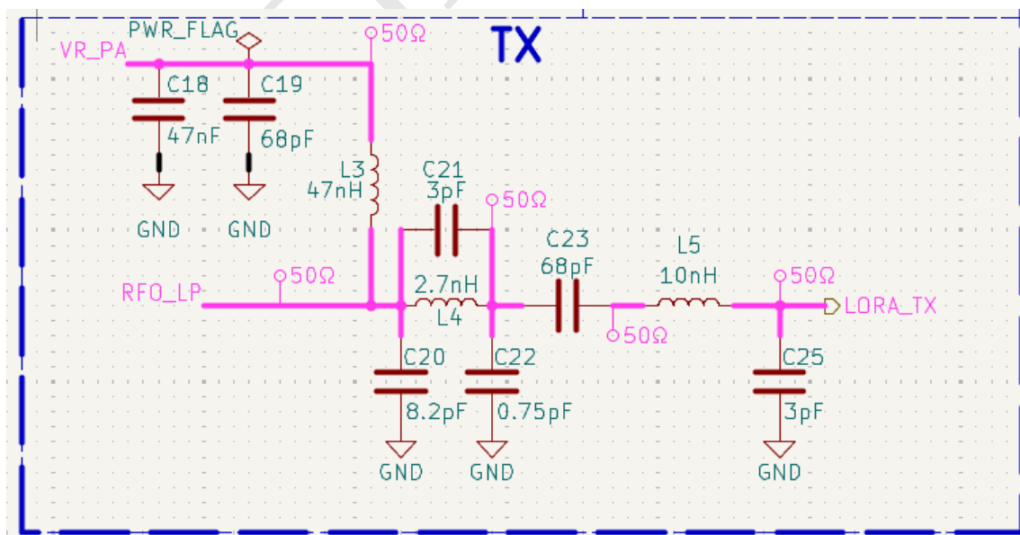
Abbildung 3.13: TX-Impedanzanpassung
