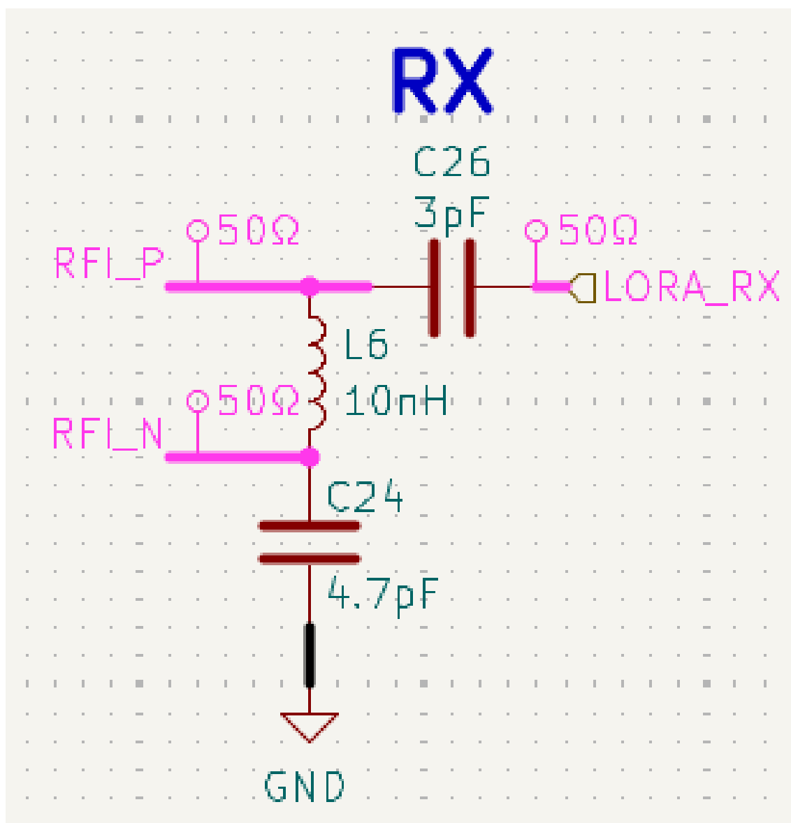
Abbildung 3.14: RX-Impedanzanpassung
