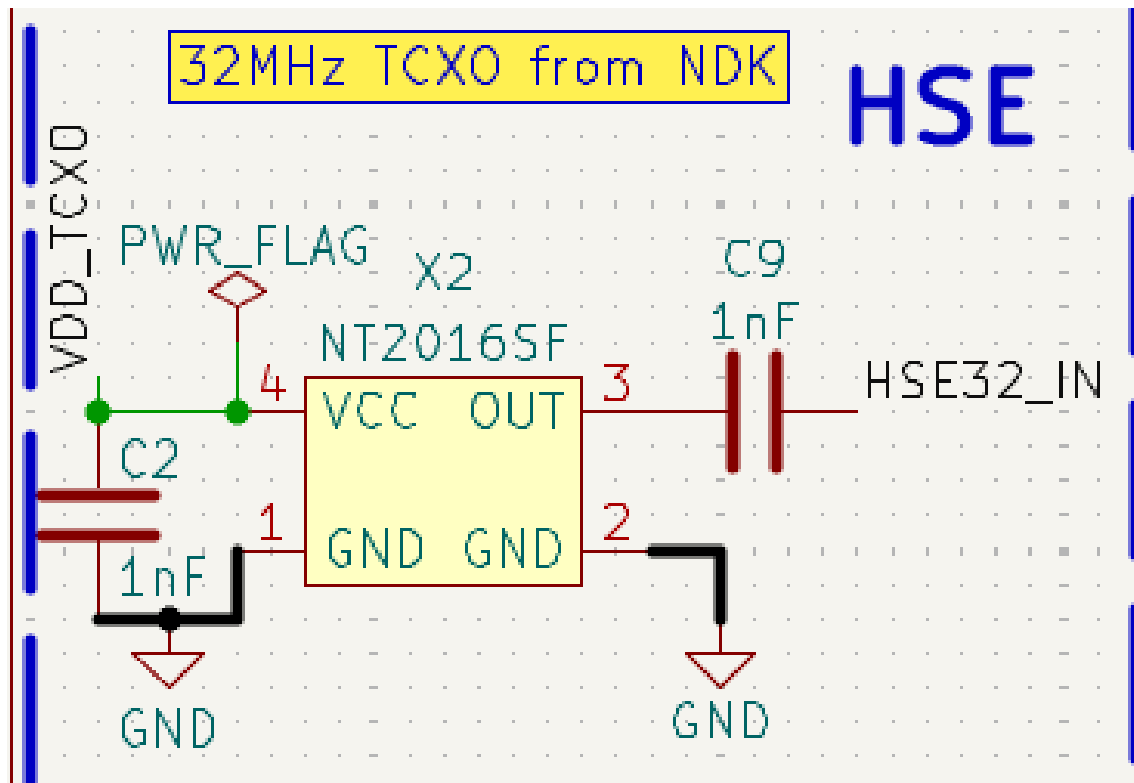
Abbildung 3.11: Taktversorgung mit HSE
