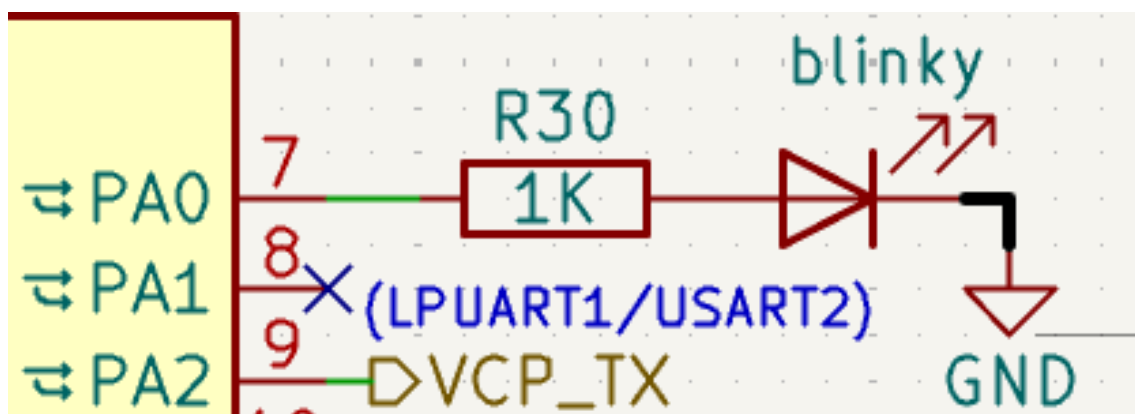
Abbildung 3.19: Status-LED
