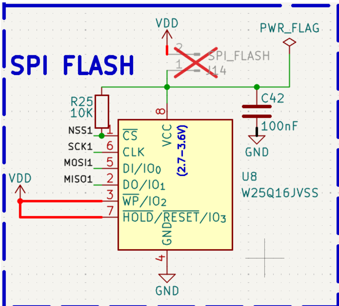
Abbildung 3.18: SPI-Flash-Speicher
