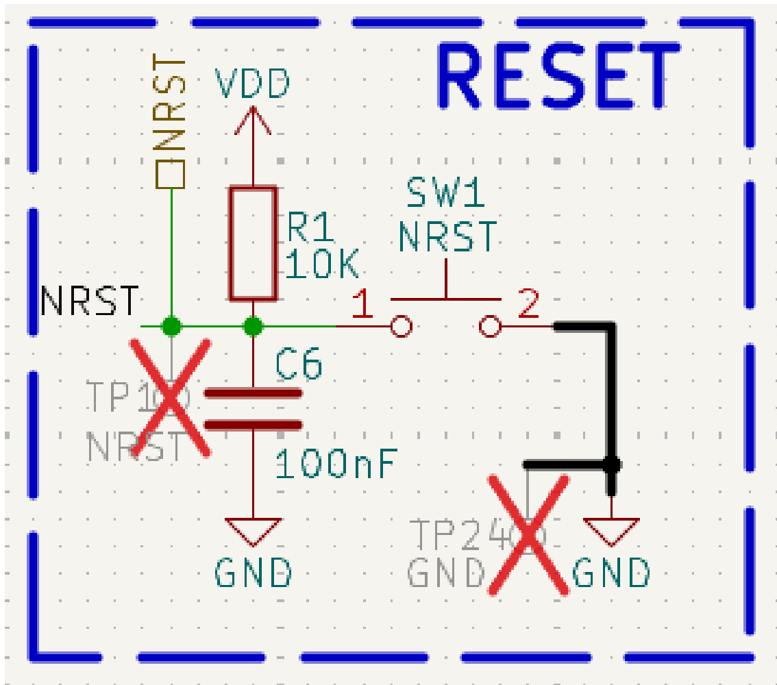
Abbildung 3.16: MCU-Reset-Schaltung
