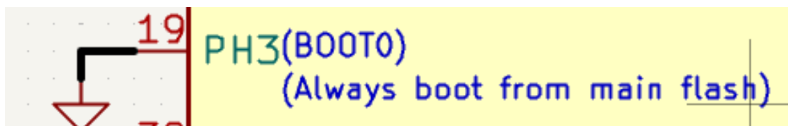
Abbildung 3.17: BOOT0-Konfiguration
