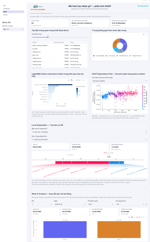
Hình 6.16: Trang 2 của ứng dụng, giải thích dự báo bằng SHAP.
