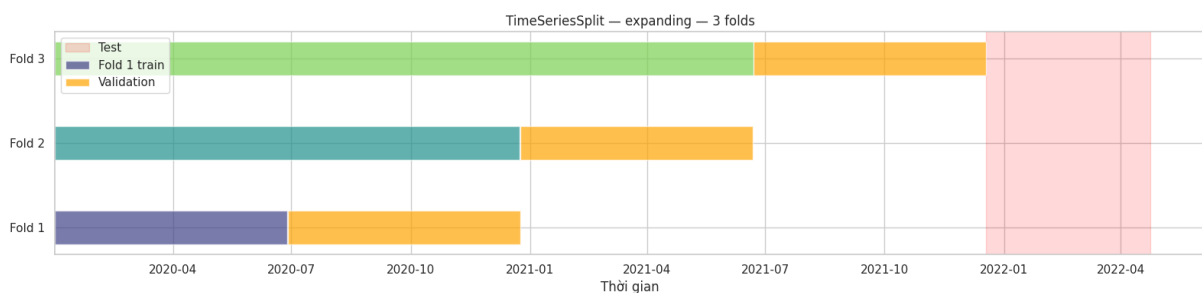
Hình 6.9: (Trích xuất từ Notebook 02_split_time_series.ipynb) Cách chia dữ liệu theo trục thời gian: tập test niêm phong tách ra từ phần cuối, phần Phát triển còn lại chia thành ba fold theo cửa sổ mở rộng.
