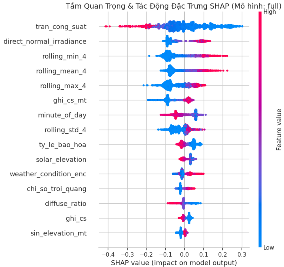
Hình 6.13: (Trích xuất từ Notebook 08_explainable_ai.ipynb) Biểu đồ beeswarm. Mỗi điểm là một dòng dữ liệu; vị trí ngang là giá trị SHAP, màu là độ lớn của chính đặc trưng đó.
