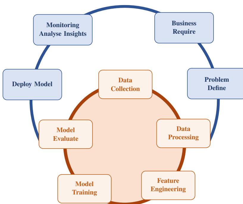
Hình 7.1: Vòng đời học máy, giữ nguyên nhữn tiếng Anh của tài liệu gốc. Nguồn: Data Version Control [24].
