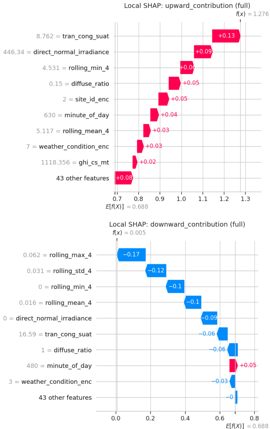
Hình 6.14: (Trích xuất từ Notebook 08_explainable_ai.ipynb) Biểu đồ thác cho hai dự báo tương phản. Trên: trường hợp các đặc trưng cùng đẩy dự báo lên. Dưới: trường hợp cùng kéo xuống.
