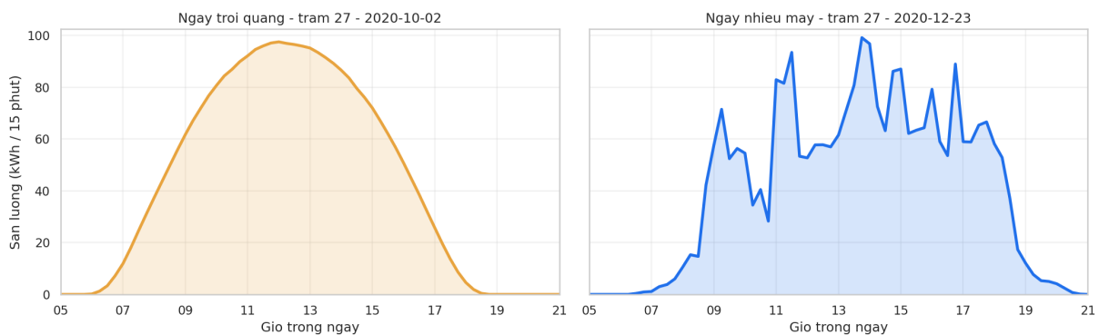
Hình 6.6: (Trích xuất từ Notebook 02_EDA.ipynb ) Sản lượng theo bước 15 phút tại trạm 27, hai ngày dùng chung thang trục tung. Trái: ngày trời quang 02/10/2020, độ gấp 0,0031. Phải: ngày nhiều mây 23/12/2020, độ gấp 0,0926. Trục hoành là giờ trong ngày, cắt trong khoảng 5–21 giờ vì ngoài khoảng đó sản lượng bằng 0. Số đo của hai ngày kiểm chứng được bằng srcs/05_machine_learning/kiem_chung_bao_cao_v4.py , mục 11.
