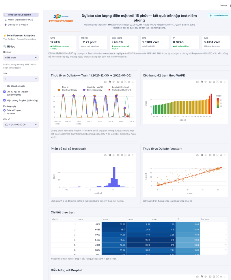
Hình 6.15: Trang 1 của ứng dụng, giám sát chuỗi thời gian theo trạm.
