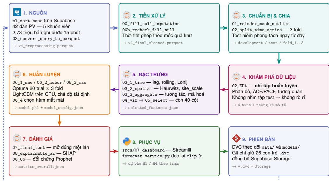
Hình 6.4: Chín bước của quy trình học máy, xếp ba hàng ba cột và đọc theo mũi tên. Hàng trên chạy từ trái sang phải là bước 1, 2, 3; hàng giữa chạy ngược từ phải sang trái là 4, 5, 6; hàng dưới lại chạy từ trái sang phải là 7, 8, 9. Dòng cuối mỗi ô ghi tệp kết quả mà bước đó sinh ra. Mũi tên nét đứt từ bước 9 vòng về bước 1 là khâu quản lý phiên bản áp lại lên tệp nguồn.
