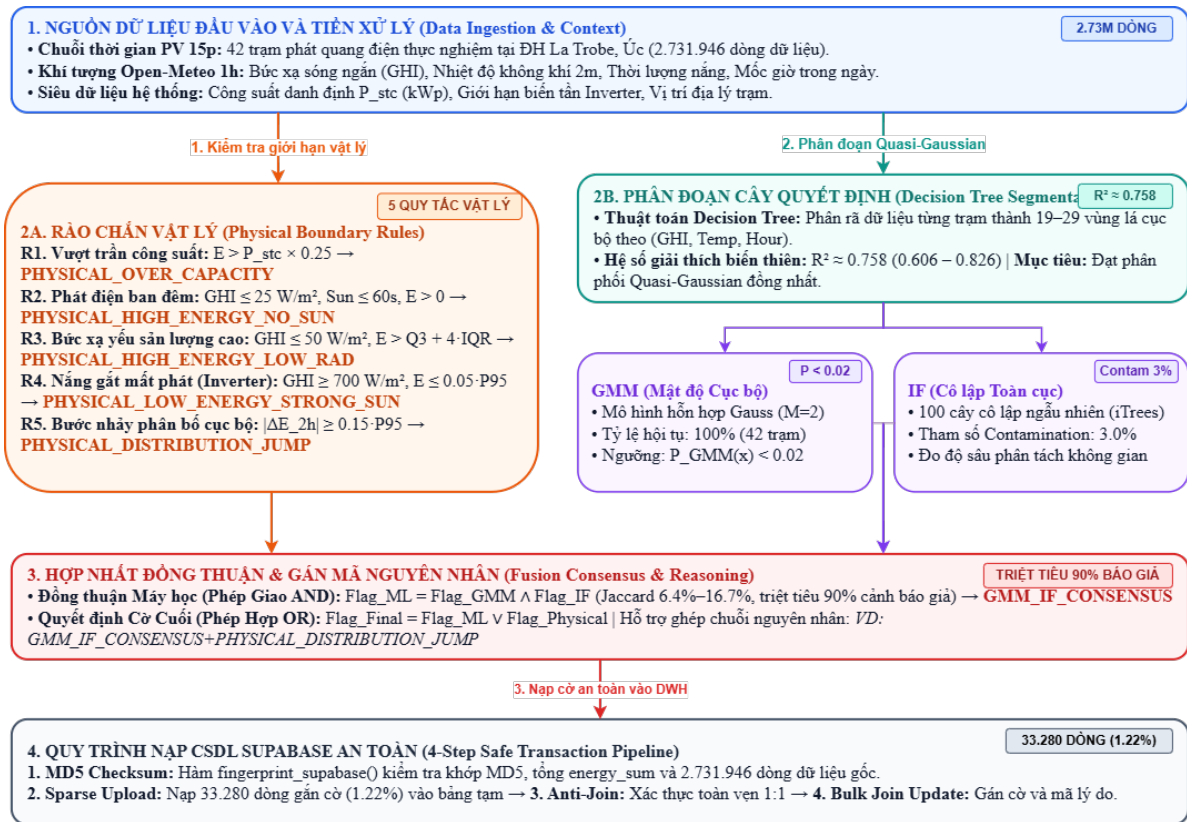
Hình 4.1: Sơ đồ kiến trúc mô hình phân lớp lai GMM–IF và ràng buộc vật lý kết hợp quy trình 4 bước nạp cơ sở an toàn vào Supabase DWH.
