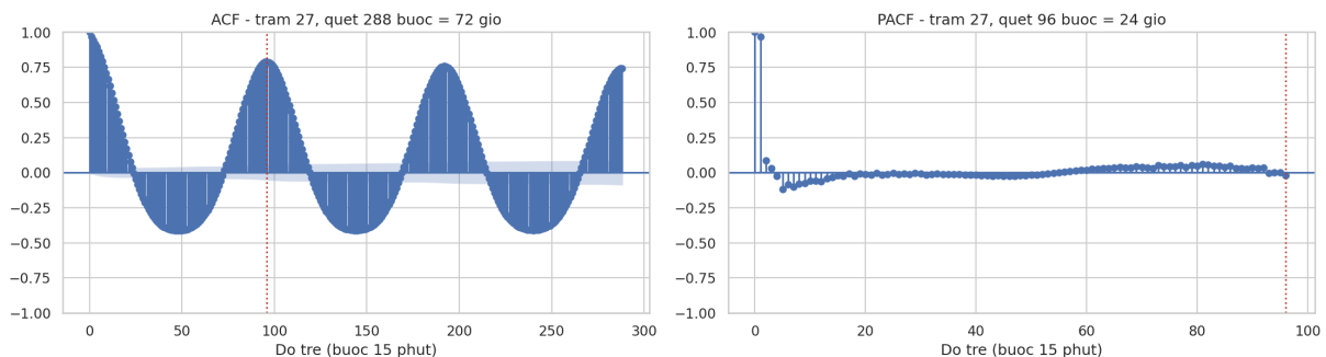
Hình 6.7: (Trích xuất từ Notebook 02_EDA.ipynb) Trái: ACF quét 288 bước = 72 giờ. Phải: PACF quét 96 bước = 24 giờ. Vạch đỏ chấm là mốc 96 bước.
