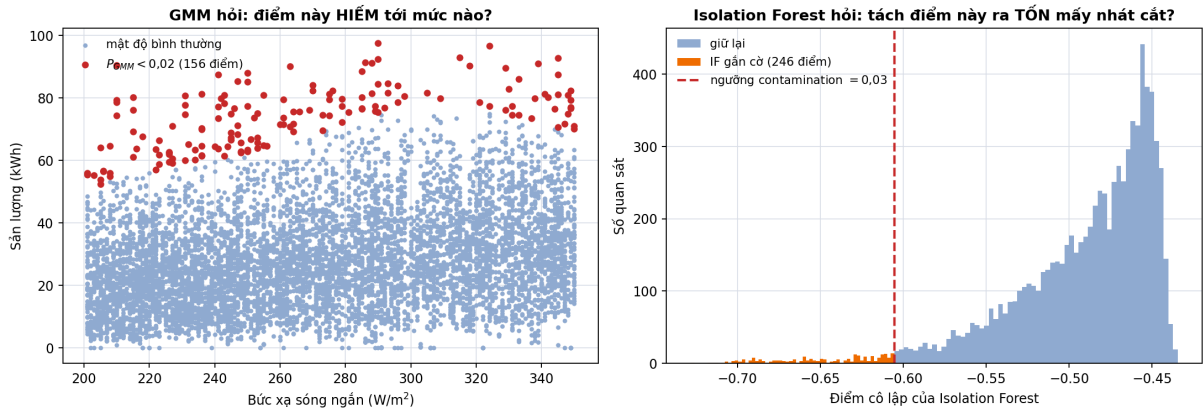
Hình 6.1: (Trích xuất từ Notebook 05d_thuc_nghiem_rao_chan_vat_ly.ipynb) Hai nguyên lý chạy trên dữ liệu thật của dự án: trạm 27, dải bức xạ 201–350 W/m 2 , 8.176 quan sát. Trái: GMM hai thành phần, điểm đỏ là các quan sát có mật độ tương đối P_{\text{GMM}} < 0,02 . Phải: phân bố điểm cô lập của Isolation Forest (100 cây), phần cam là vùng bị cắt theo \text{contamination} = 0,03 .
