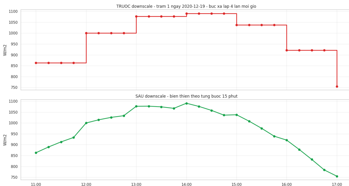
Hình 8.10: (Trích xuất từ Notebook 03_2_features_spatial.ipynb) Bức xạ tại trạm 1, ngày 19/12/2020, từ 11 giờ đến 17 giờ. Trên: dữ liệu gốc theo giờ, mỗi giá trị lặp bốn lần nên đường đi thành bậc thang. Dưới: sau khi hạ độ hạt, đường biến thiên theo từng bước 15 phút.
