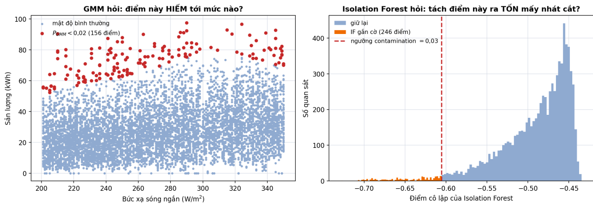
Hình 8.1: (Trích xuất từ Notebook 05d_thuc_nghiem_rao_chan_vat_ly.ipynb) Hai nguyên lý chạy trên dữ liệu thật của dự án: trạm 27, dải bức xạ 201–350 W/m 2 , 8.176 quan sát. Trái: GMM hai thành phần, điểm đỏ là các quan sát có mật độ tương đối P_{GMM} < 0,02 . Phải: phân bố điểm cô lập của Isolation Forest (100 cây), phần cam là vùng bị cắt theo \text{contamination} = 0,03 .
