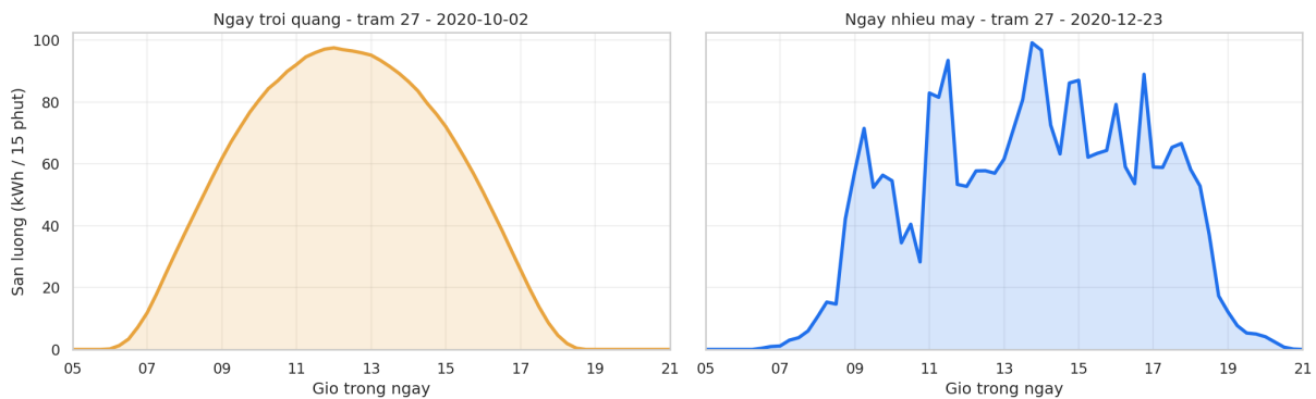
Hình 8.6: (Trích xuất từ Notebook 02_EDA.ipynb ) Sản lượng theo bước 15 phút tại trạm 27, hai ngày dùng chung thang trục tung. Trái: ngày trời quang 02/10/2020, độ gập 0,0031. Phải: ngày nhiều mây 23/12/2020, độ gập 0,0926. Trục hoành là giờ trong ngày, cắt trong khoảng 5–21 giờ vì ngoài khoảng đó sản lượng bằng 0. Số đo của hai ngày kiểm chứng được bằng srcs/05_machine_learning/kiem_chung_bao_cao_v4.py , mục 11.
