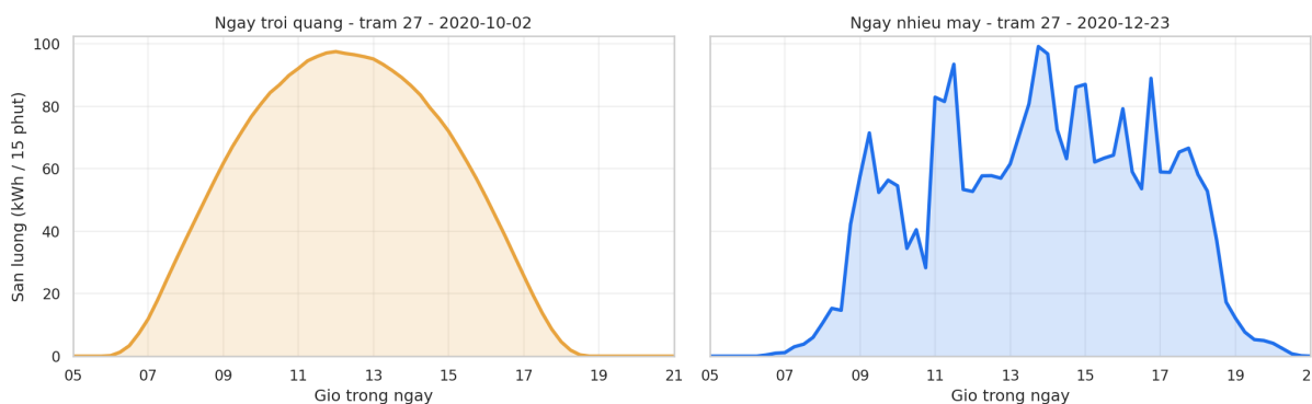
Hình 8.6: (Trích xuất từ Notebook 02_EDA.ipynb ) Sản lượng theo bước 15 phút tại trạm 27, hai ngày dùng chung thang trục tung. Trái: ngày trời quang 02/10/2020, độ gấp 0,0031. Phải: ngày nhiều mây 23/12/2020, độ gấp 0,0926. Trục hoành là giờ trong ngày, cắt trong khoảng 5–21 giờ vì ngoài khoảng đó sản lượng bằng 0. Số đo của hai ngày kiểm chứng được bằng srcs/05_machine_learning/kiem_chung_bao_cao_v4.py , mục 11.
