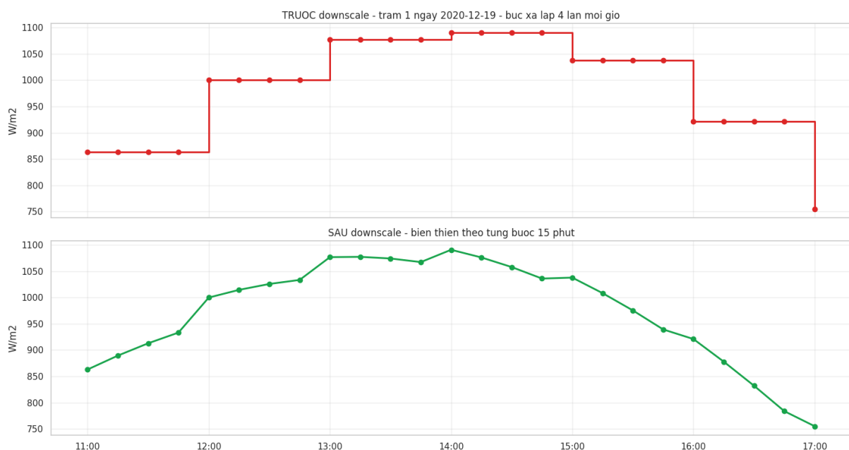
Hình 8.11: (Trích xuất từ Notebook 03_2_features_spatial.ipynb) Bức xạ tại trạm 1, ngày 19/12/2020, từ 11 giờ đến 17 giờ. Trên: dữ liệu gốc theo giờ, mỗi giá trị lặp bốn lần nên đường đi thành bậc thang. Dưới: sau khi hạ độ hạt, đường biến thiên theo từng bước 15 phút.
