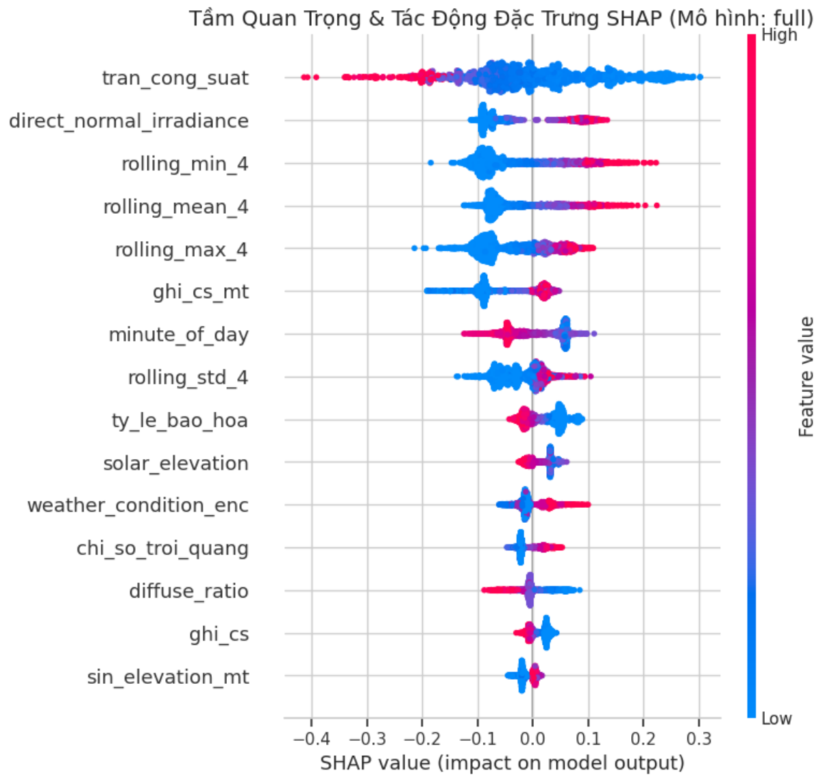
Hình 8.13: (Trích xuất từ Notebook 08_explainable_ai.ipynb) Biểu đồ beeswarm. Mỗi điểm là một dòng dữ liệu; vị trí ngang là giá trị SHAP, màu là độ lớn của chính đặc trưng đó.
