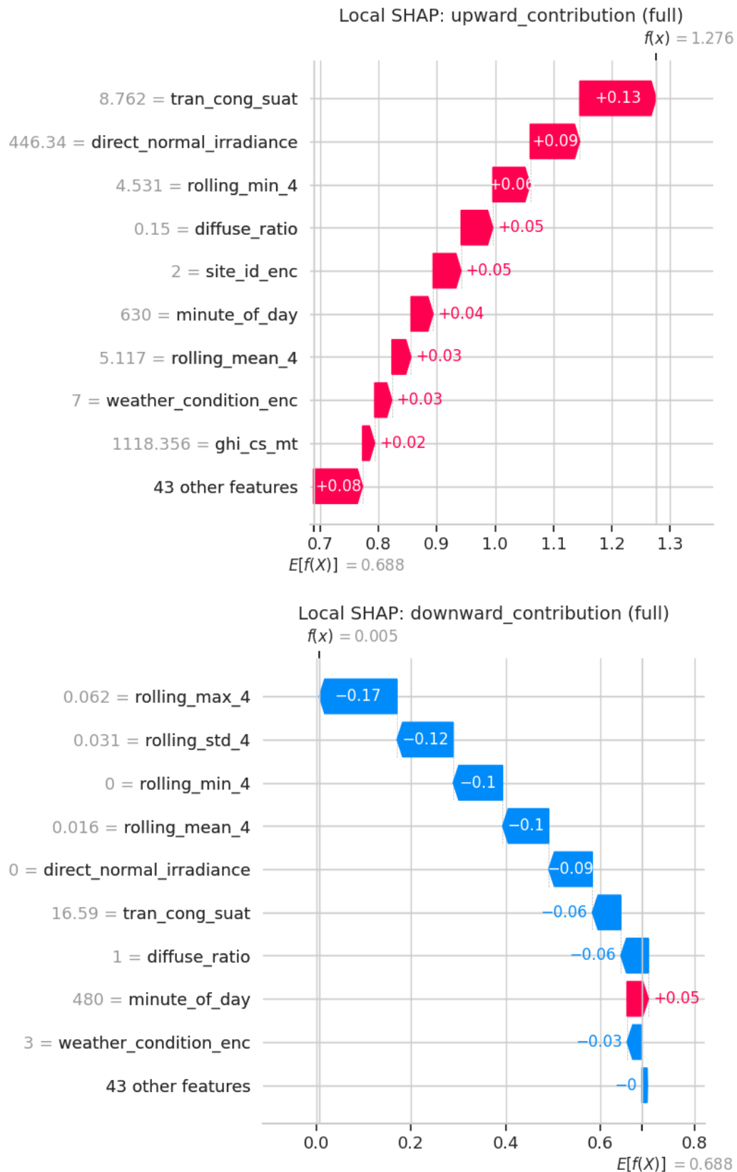
Hình 8.14: (Trích xuất từ Notebook 08_explainable_ai.ipynb) Biểu đồ thác cho hai dự báo tương phản. Trên: trường hợp các đặc trưng cùng đẩy dự báo lên. Dưới: trường hợp cùng kéo xuống.
