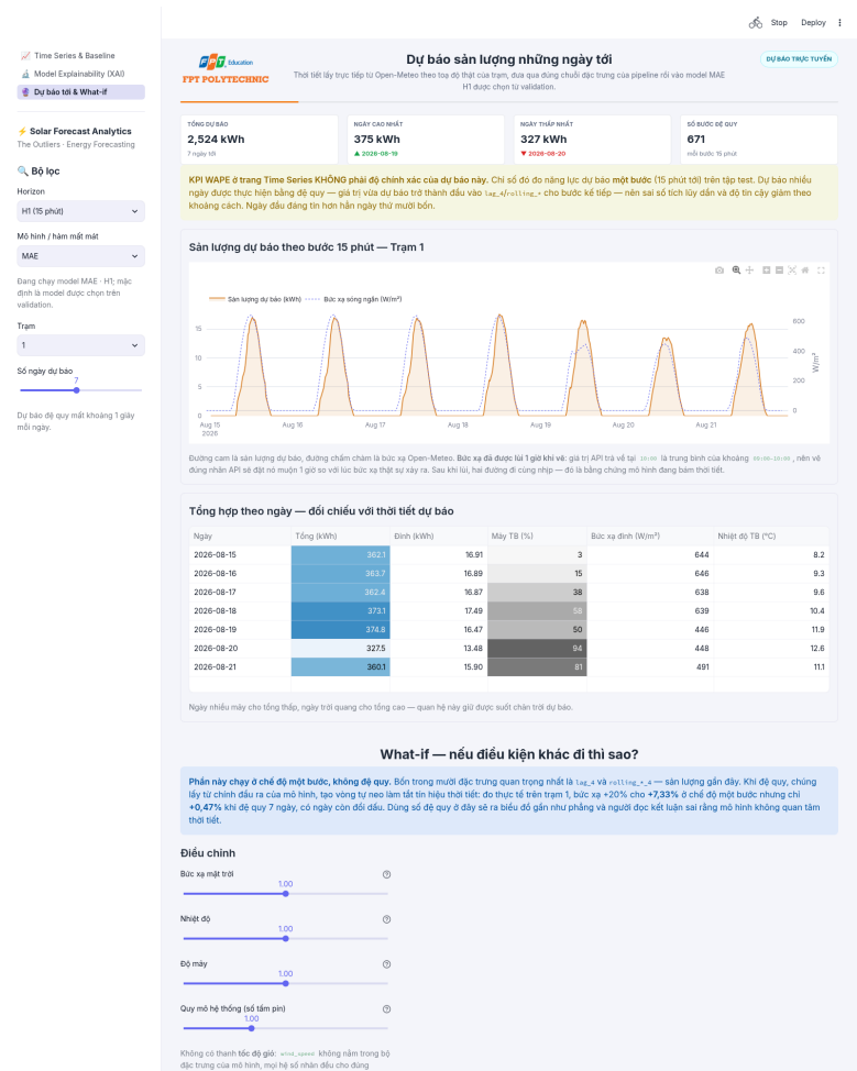
Hình 6.17: Trang 3 của ứng dụng, dự báo và phân tích giả định.
