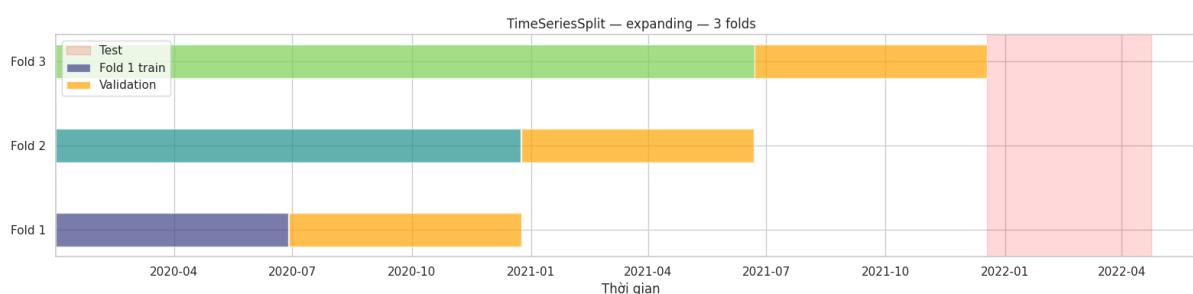
Hình 6.9: (Trích xuất từ Notebook 02_split_time_series.ipynb ) Cách chia dữ liệu theo trục thời gian: tập test niêm phong tách ra từ phần cuối, phần Phát triển còn lại chia thành ba fold theo cửa sổ mở rộng.
