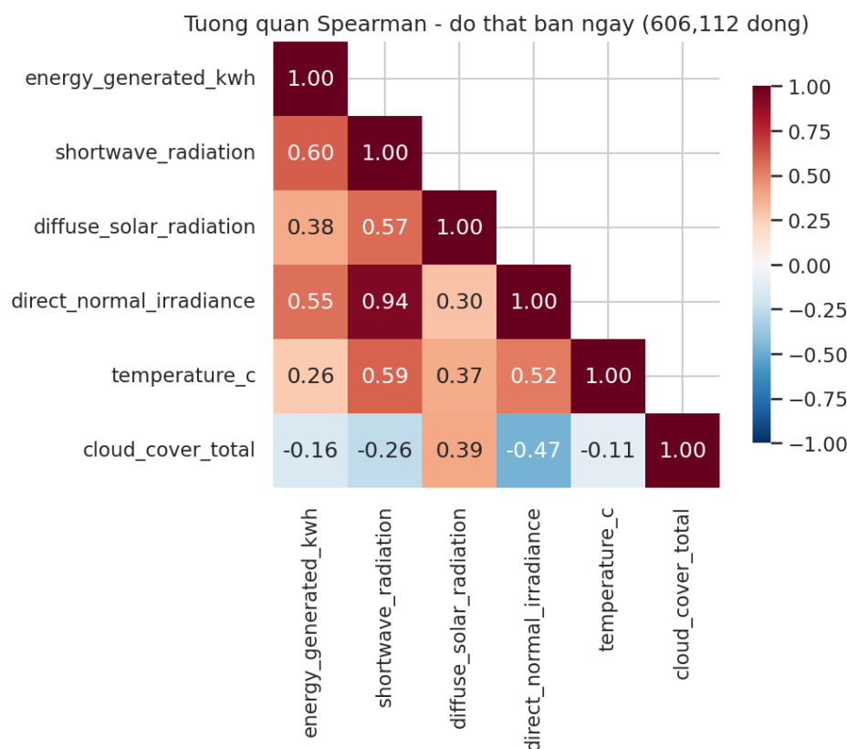
Hình 6.8: (Trích xuất từ Notebook 02_EDA.ipynb) Ma trận tương quan Spearman trên 606.112 dòng đo thật ban ngày.
