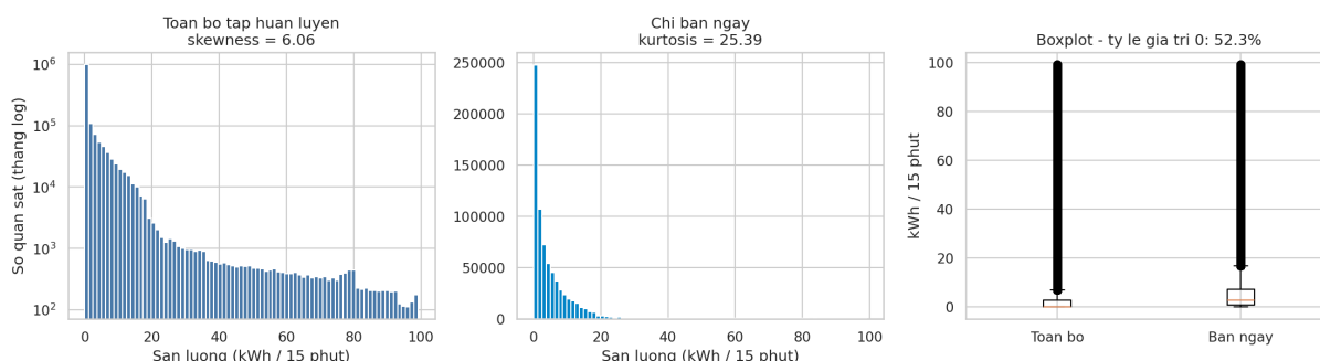
Hình 6.5: (Trích xuất từ Notebook 02_EDA.ipynb) Trái: histogram toàn bộ tập huấn luyện, trục tung thang loga. Giữa: chỉ ban ngày. Phải: boxplot đối chiếu hai phạm vi.
