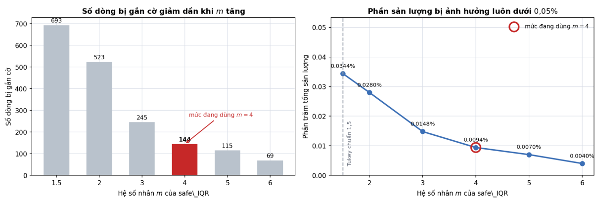
Hình 6.2: (Trích xuất từ Notebook 05d_thuc_nghiem_rao_chan_vat_ly.ipynb ) Quét hệ số nhân m của safe_IQR qua sáu mức. Trái: số dòng bị gắn cờ. Phải: phần sản lượng bị ảnh hưởng, trực tung dừng ở 0,05%.
