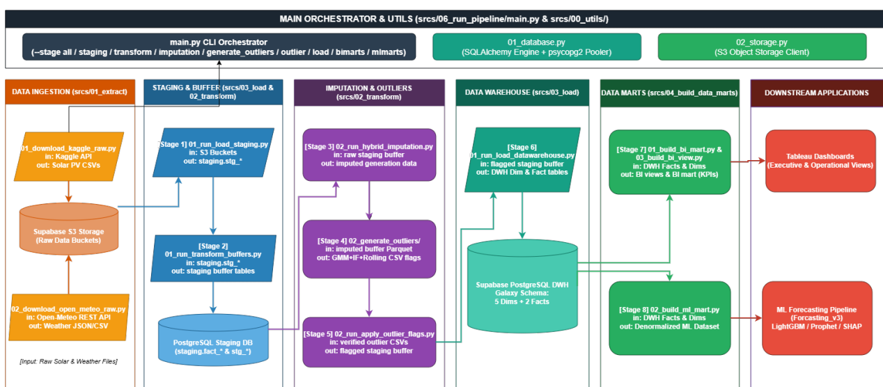
Hình 3.1: Sơ đồ luồng thực thi quy trình xử lý dữ liệu tự động
