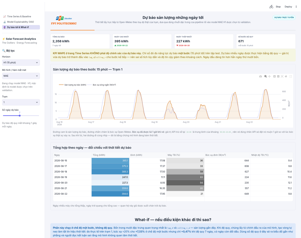
Hình 6.15: Giao diện Trang 3: Dự báo và phân tích giả định (What-If Analysis)
