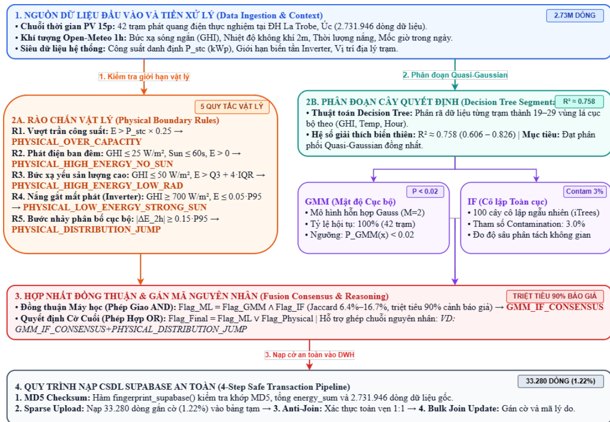
Hình 4.1: Sơ đồ kiến trúc mô hình phân lớp lai GMM–IF và rào chắn vật lý kết hợp quy trình 4 bước nạp cơ sở an toàn vào Supabase DWH.
