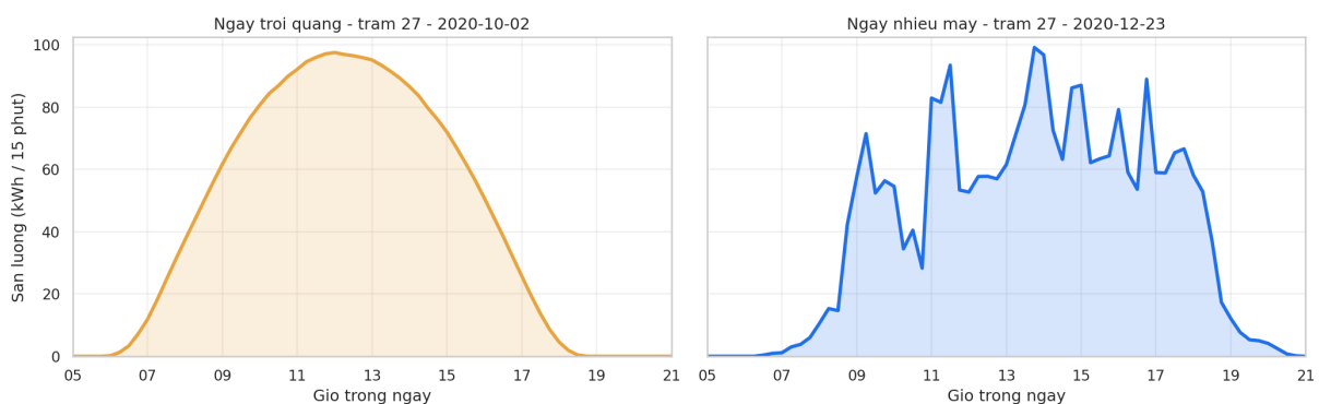
Hình 8.6: (Trích xuất từ Notebook 02_EDA.ipynb) Sản lượng theo bước 15 phút tại trạm 27, hai ngày dùng chung thang trục tung. Trái: ngày trời quang 02/10/2020, độ gấp 0,0031. Phải: ngày nhiều mây 23/12/2020, độ gấp 0,0926. Trục hoành là giờ trong ngày, cắt trong khoảng 5–21 giờ vì ngoài khoảng đó sản lượng bằng 0. Số đo của hai ngày kiểm chứng được bằng srcs/05_machine_learning/kiem_chung_bao_cao_v4.py , mục 11.
