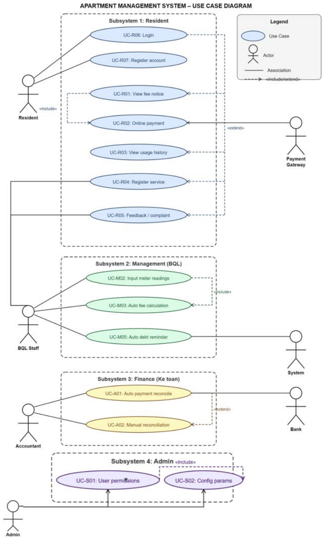
Hình 1 Usecase Diagram
