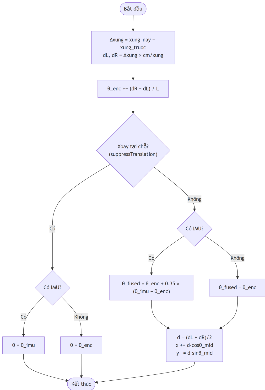
Hình 3.12 — Lưu đồ cập nhật odometry
