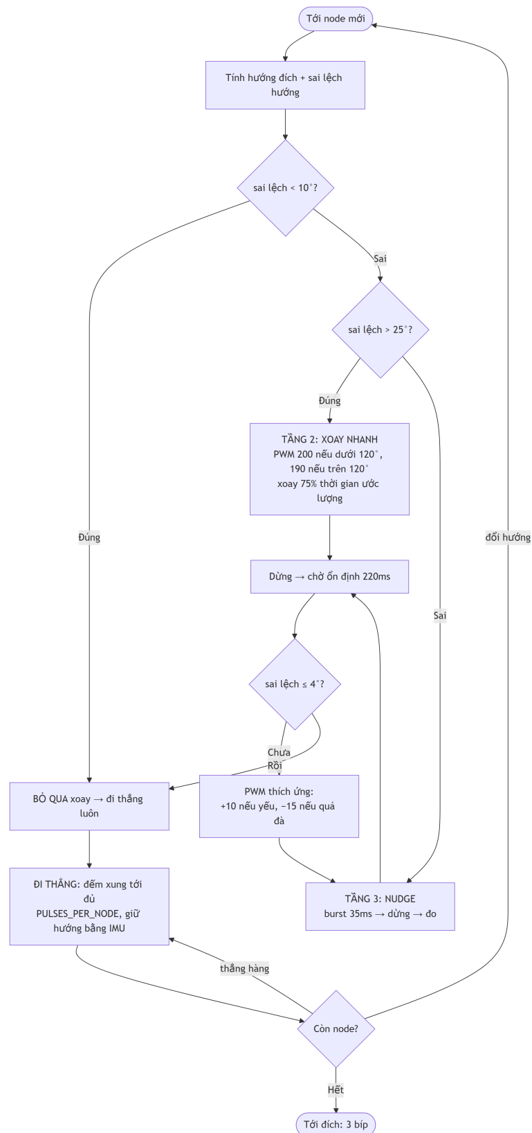
Hình 3.13 — Lưu đồ điều hướng node 3 tầng xoay
