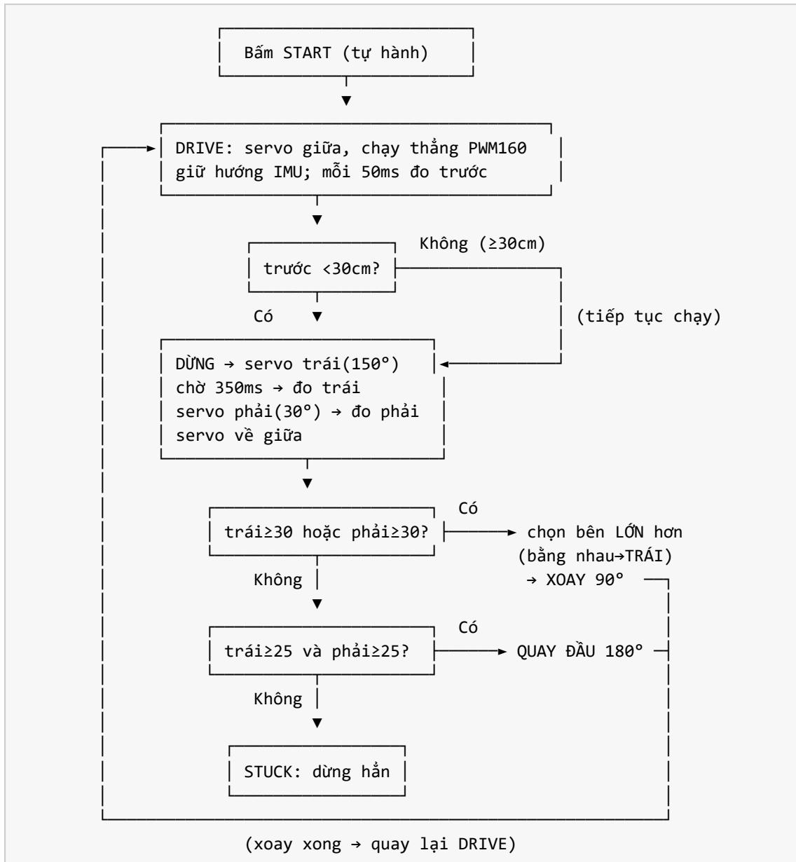
Hình 3.17 — Lưu đồ giải thuật chế độ tự hành né vật cản
