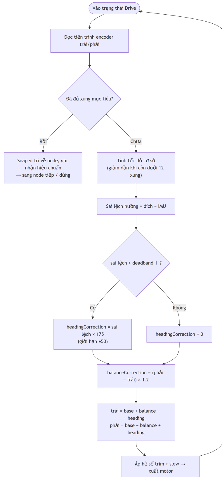
Hình 3.14 — Lưu đồ chương trình con đi thẳng
