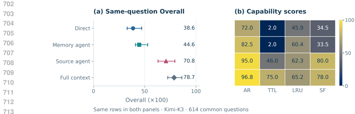
图 4: 同模型完整上下文参照覆盖的 n=614 题上的问题对齐 (Kimi-K3 作答; 官方宏平均评分器)。(a) 带边缘 95% bootstrap 区间的 Overall 分数; 原文读取方式低于参照 7.9 个百分点 [95% CI -11.9, -3.9]。(b) 域画像: 参照的领先集中在 TTL, 而原文读取方式在 AR、LRU、SF 上与参照持平或反超。
