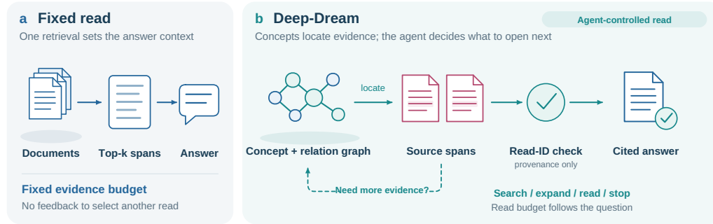
图 1: 寻址与加载分离。固定检索一次性决定读什么; Deep-Dream 先沿概念链接定位候选源文本 (寻址), 再由智能体在预算内读取 (加载)、验证或停止。
