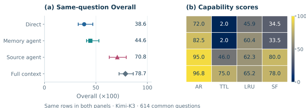
图 4: 同模型完整上下文参照覆盖的 n=614 题上的同题对齐 (Kimi-K3 作答; 官方宏平均评分器)。(a) 带边缘 95% bootstrap 区间的 Overall 分数; 原文读取方式低于参照 7.9 个百分点 [95% CI -11.9, -3.9]。(b) 域画像: 参照的领先集中在 TTL, 而原文读取方式在 AR、LRU、SF 上与参照持平或反超。
