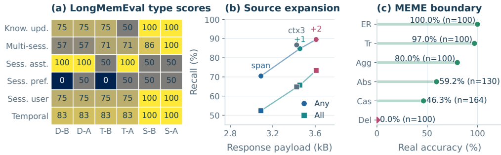
图 8: 来自冻结账本的额外定量诊断。(a) 配对 Base/Align+ 轨道的 LongMemEval 类型分数; 这些方向性样本 n=25/25/27 , 以粗略百分比显示。(b) 105 个历史错误案例上的源扩展召回对响应载荷; 这是开发诊断, 不是留出测试。(c) 带任务特定分母的 MEME 真实任务准确率, 暴露 0% 的删除边界。
