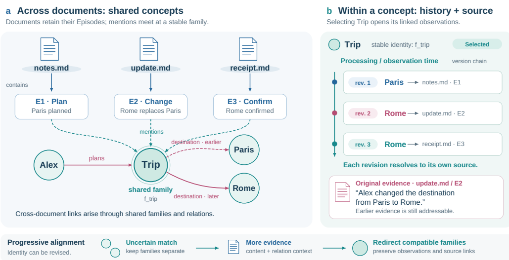
图 3: Deep-Dream 的文档优先时序概念图谱。多份文档保留各自的会话片段, 并通过共享的概念族与关系边连接。选中一个族会暴露其按观测时间排列的版本链, 以及每次修订的精确源跨度; 不确定的匹配可以先保持分离, 等到后续内容与关系上下文到达时再收敛。
