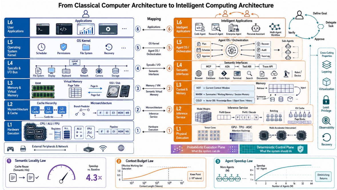
Figure 1: 计算机体系结构与模型原生计算系统之间的类比映射总览
