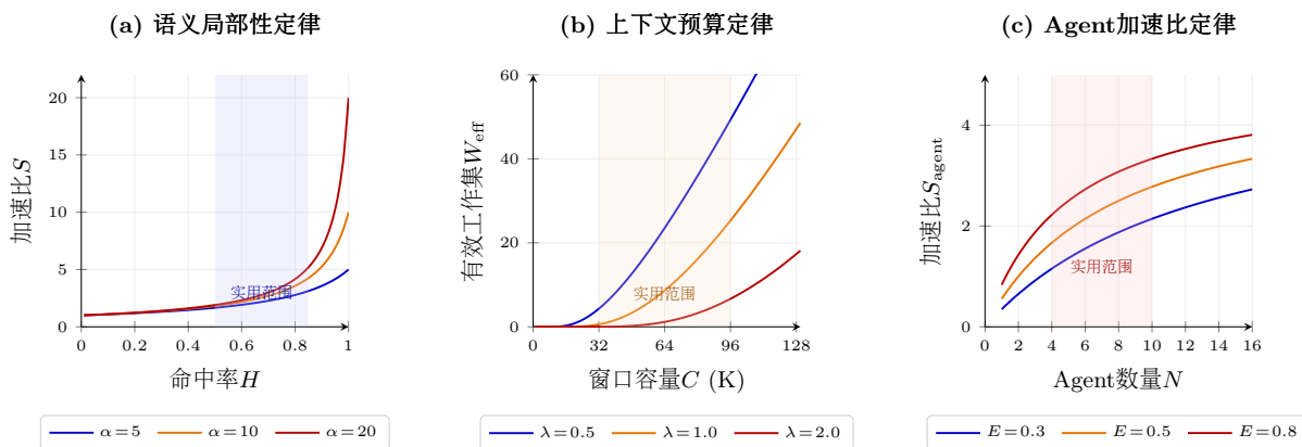
Figure 7: 三条量化定律的特征曲线。(a) 语义局部性定律: S = 1/((1 - H) + H/\alpha) 。(b) 上下文预算定律: W_{\text{eff}} = C \cdot \beta_0 e^{-\lambda C_0/C} 。(c) Agent加速比定律: S = 1/((1 - F) + F/(NE)) , 取 F = 0.8 。阴影区域为典型工作范围。
